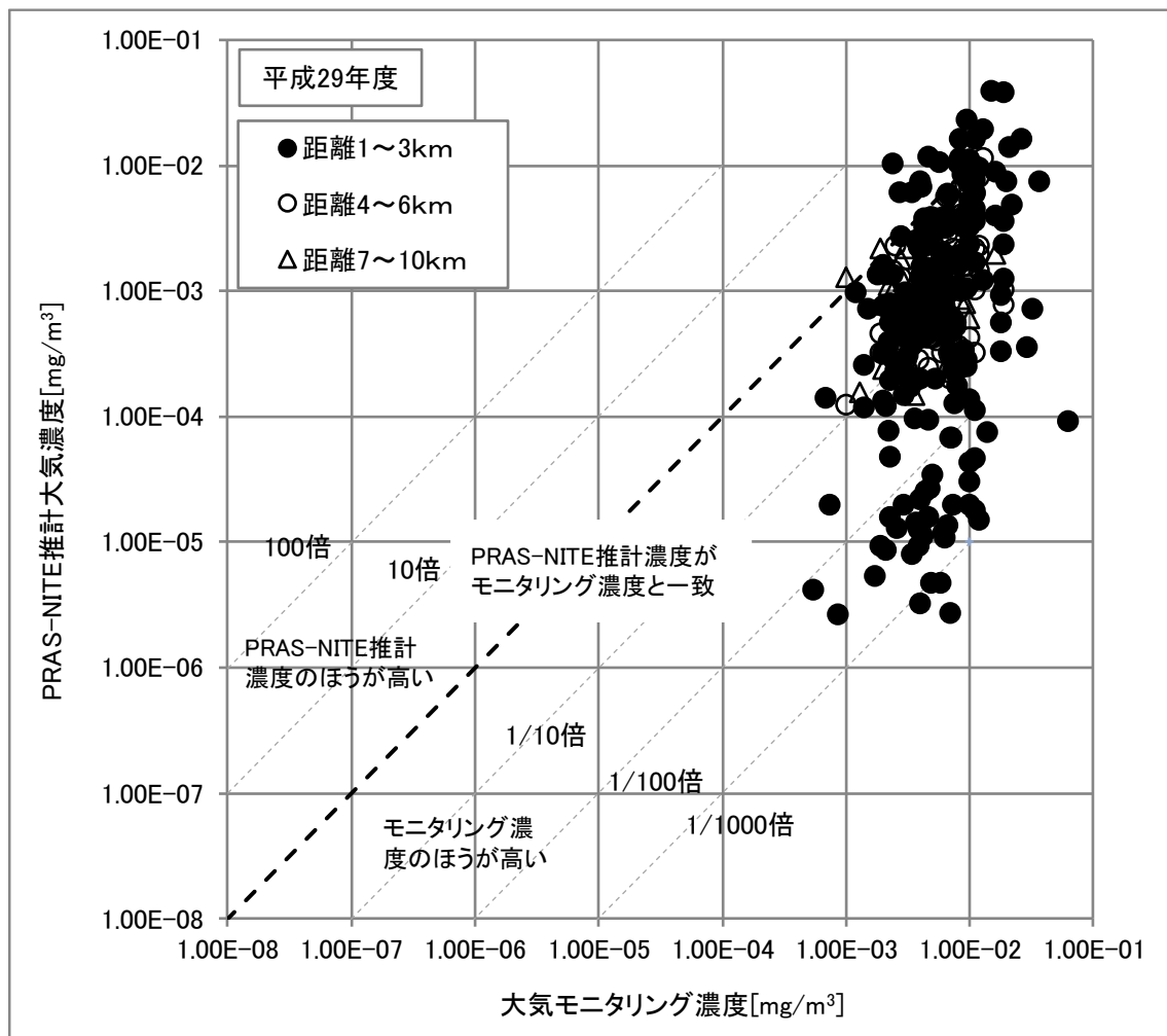
図 5 PRAS-NITE の推計大気濃度 (PRTR、平成 29 年度) と モニタリング大気濃度 (有害大気、平成 29 年度) の比較
