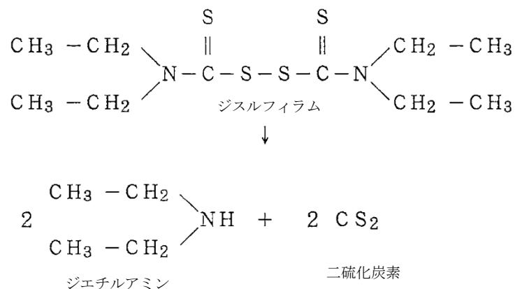
図 1-1 ジスルフィラムの生分解試験による生成物
