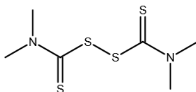
図 1-2 チウラムの構造式
