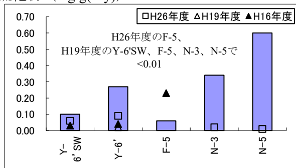
硫化物 (mg/g(dry))
