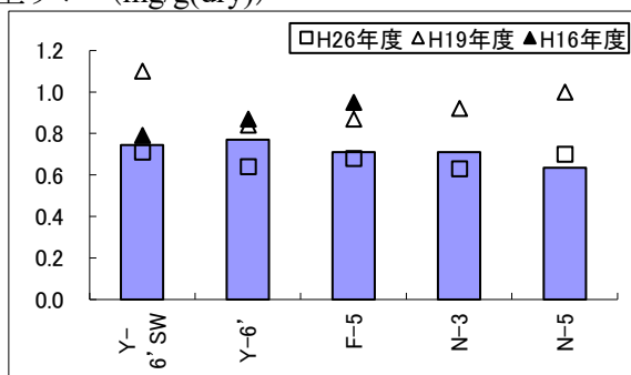
全リン (mg/g(dry))
