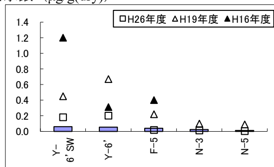
総水銀 (μg/g(dry))
