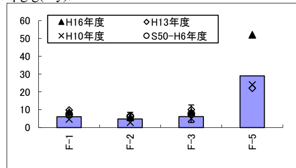
鉛 (μg/g(dry))
