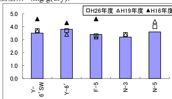
全窒素 (mg/g(dry))
