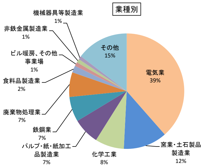
図 4 業種別の NOx 排出量内訳（総排出量：160,904 千 \text{m}^3\text{N}/\text{年} ）（令和 5 年度）
