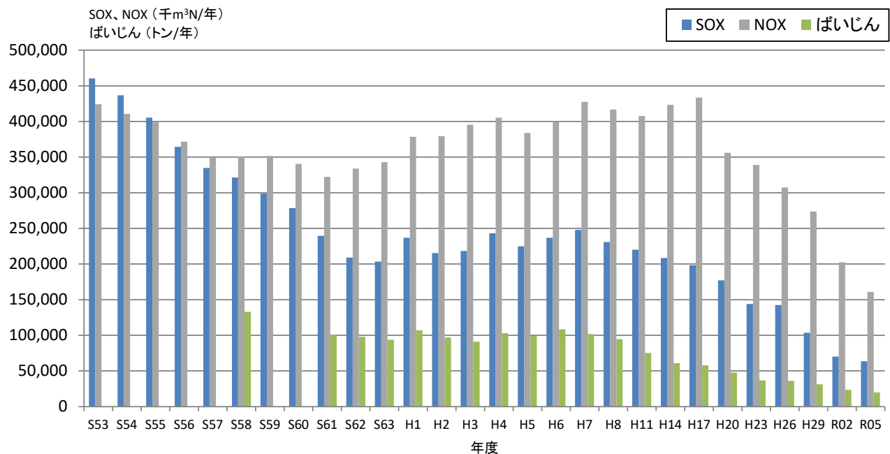
図 1 ばい煙年間排出量の推移 (令和 5 年度は暫定値)
