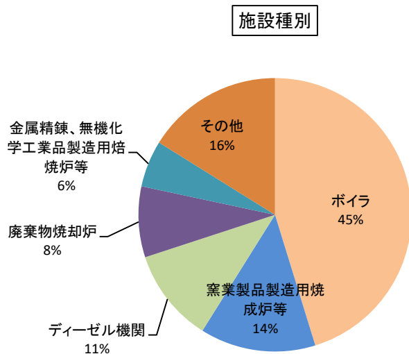
図 5 施設種別の NOx 排出量内訳（総排出量：160,904 千 \text{m}^3\text{N}/\text{年} ）（令和 5 年度）
