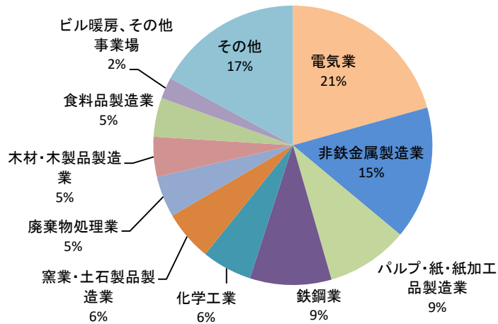
図 6 業種別のばいじん排出量内訳（総排出量：19,930 トン/年）（令和 5 年度）
