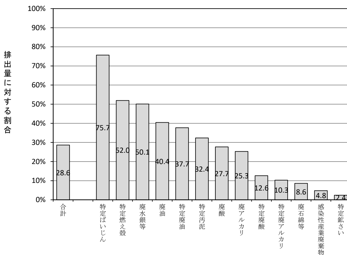
図－Ⅲ・6 特別管理産業廃棄物の種類別再生利用率（令和5年度速報値）
