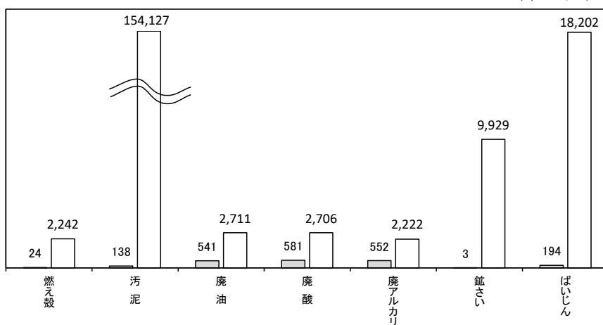
図Ⅲ・13 特別管理産業廃棄物と産業廃棄物の種類別排出量の比較（令和5年度速報値）
