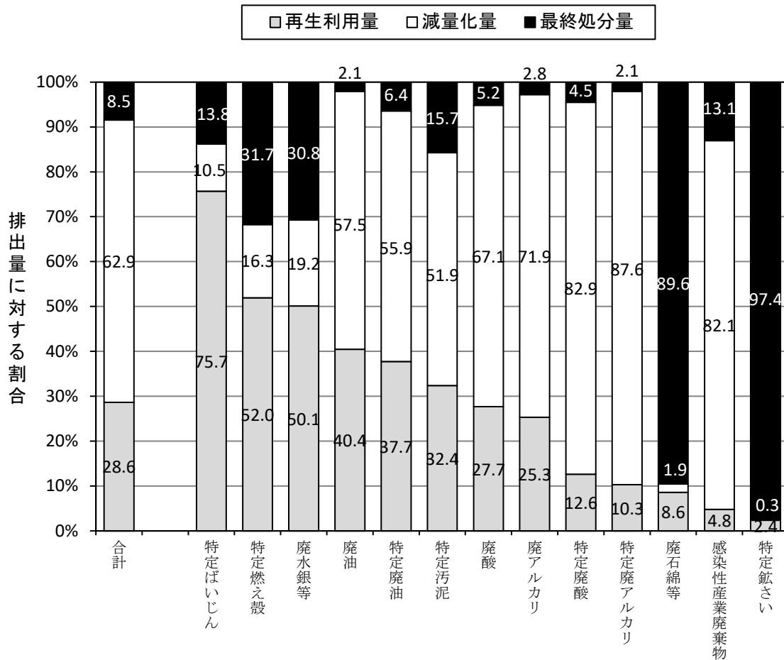
図－Ⅲ・５ 特別管理産業廃棄物の種類別の処理状況（令和５年度速報値）
