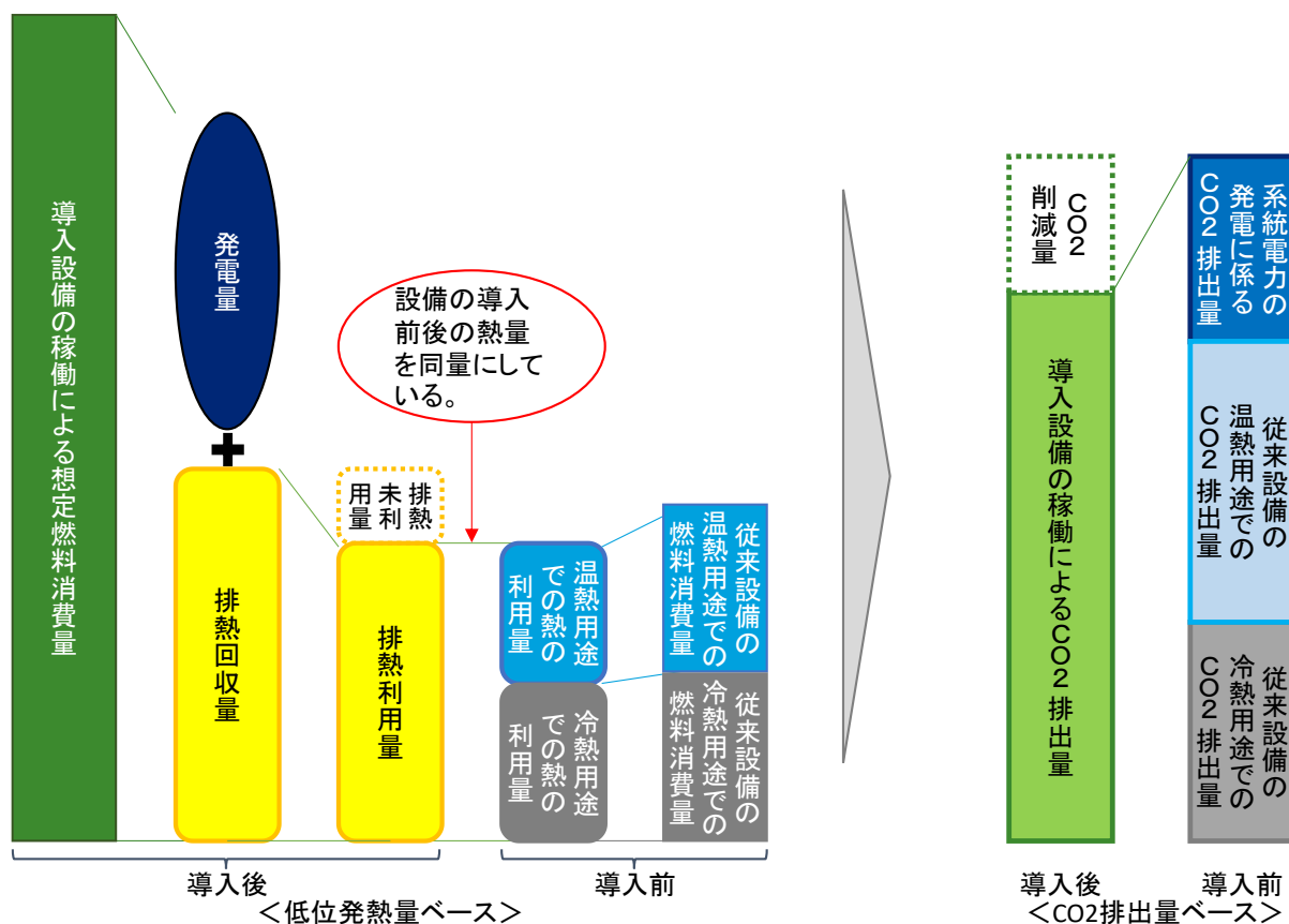
図 3 コジェネレーションや燃料電池の CO2 削減効果の考え方
