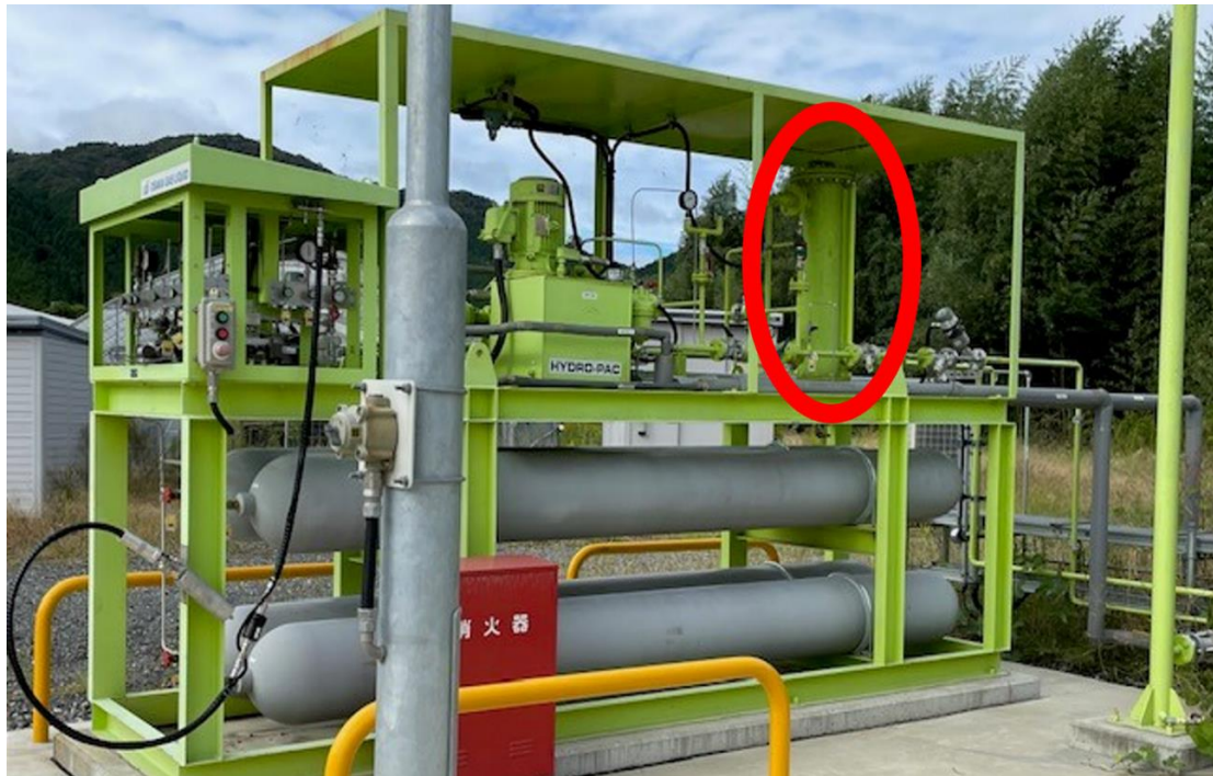
【脱湿器写真】
