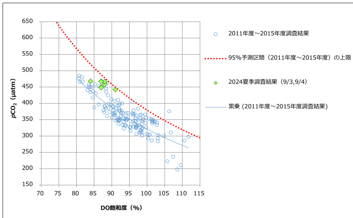
図2 p\text{CO}_2 と DO 飽和度との関係
