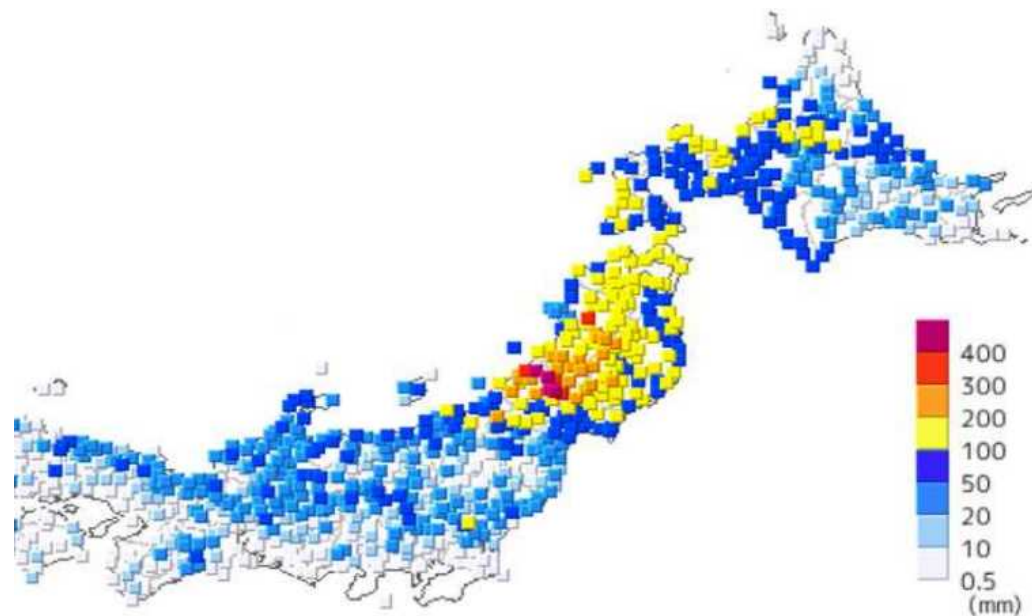
降水量の期間合計値 (7月24日～29日09時00分)
