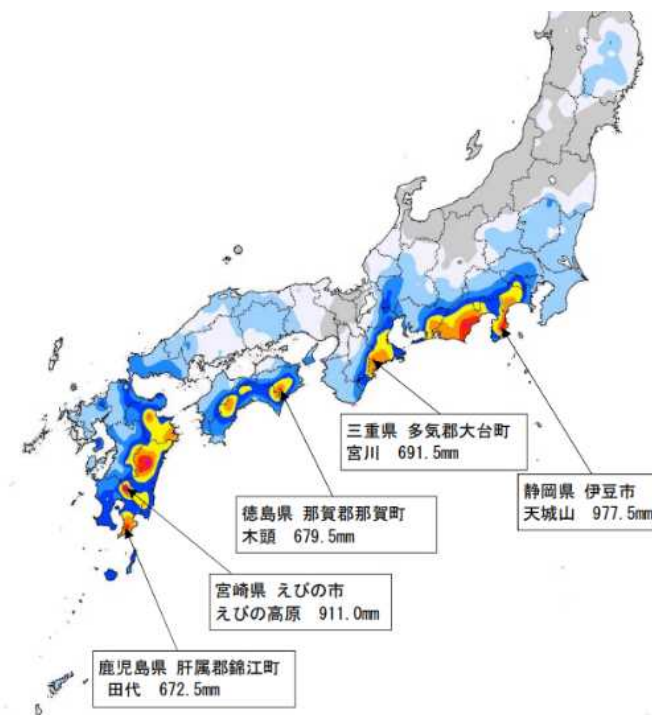
降水量の期間合計値分布図（8月27日～9月1日）
