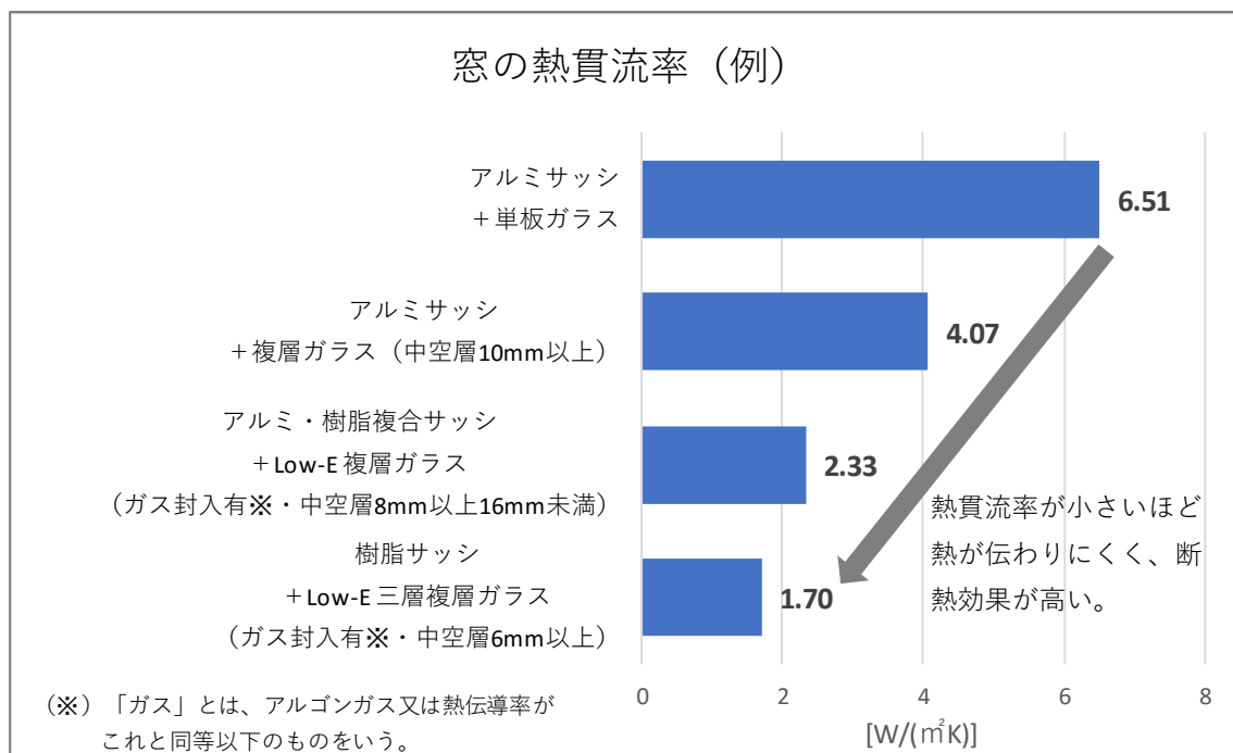
図 2 窓の断熱性能
