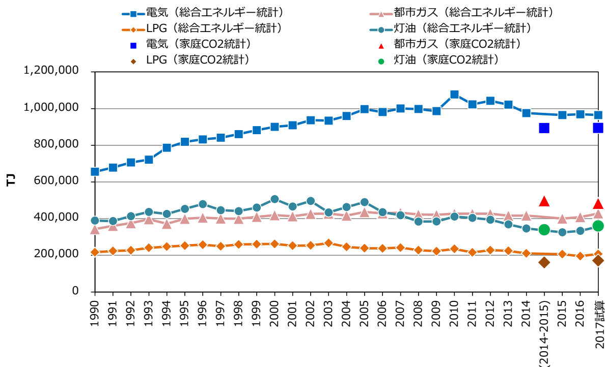
図 4.2.1 総合エネルギー統計と家庭 CO 2 統計の時系列比較
