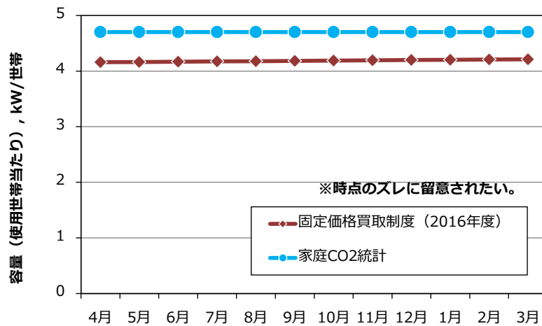
図 4.1.4 固定価格買取制度（2016 年度）と家庭 CO 2 統計（2017 年度）の比較 （使用世帯当たり太陽電池容量）
