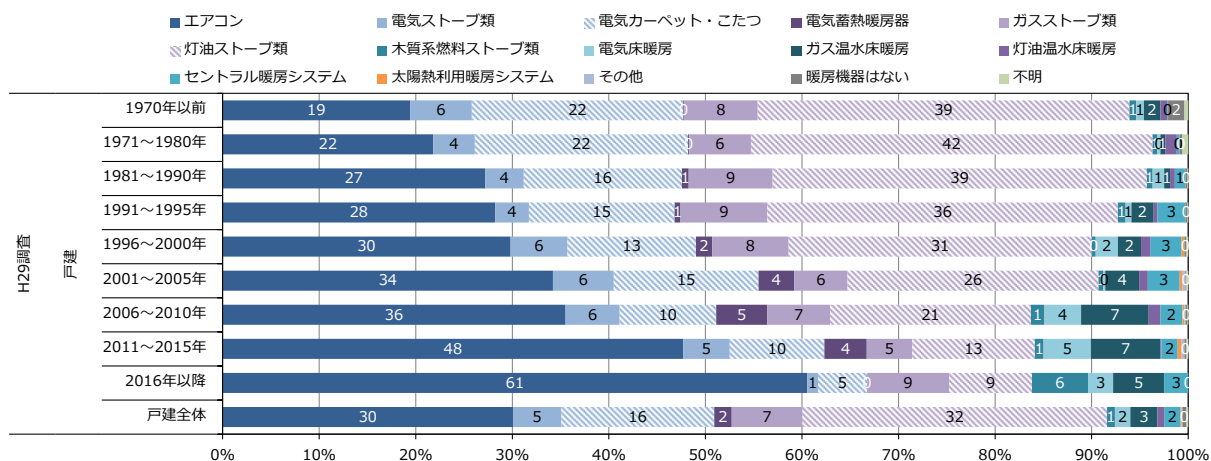
図 2.2.11 建築時期別最もよく使う暖房機器の世帯分布（戸建住宅）（平成 29 年度調査）
