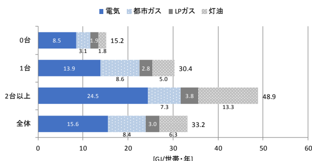
図 12 冷蔵庫の使用台数別世帯あたり年間エネルギー種別消費量
