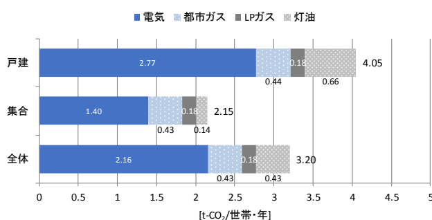
図 3 建て方別世帯あたり年間 CO 2 排出量
