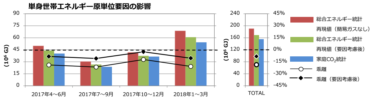
図 2.2.31 総合エネルギー統計試算値と家庭 CO 2 統計の四半期別乖離 (LP ガス) (簡易ガス要因の影響)
