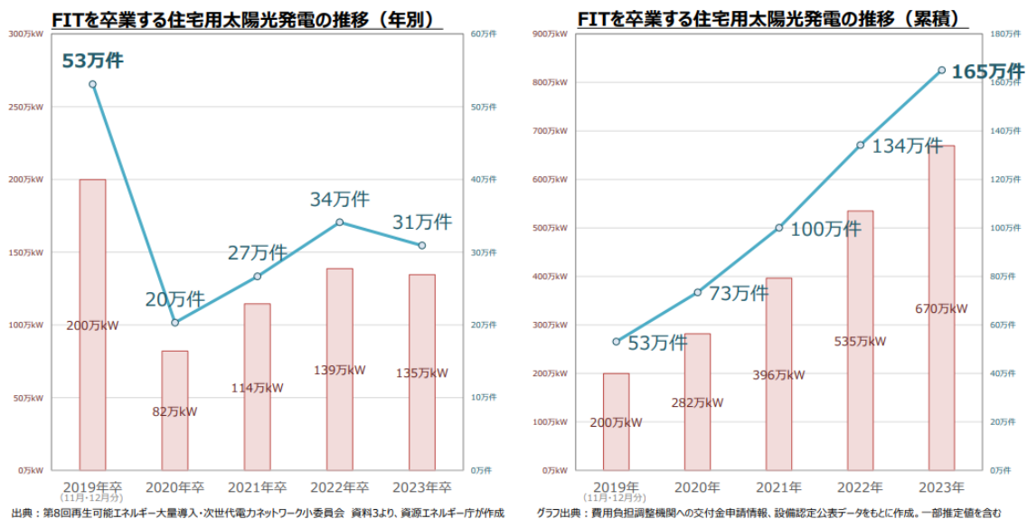
図 4.1.1 固定買取価格制度が終了する世帯の推移
