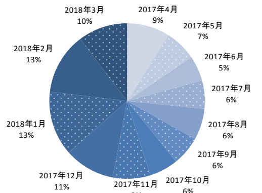
図8 世帯当たり月別 CO 2 排出構成比
