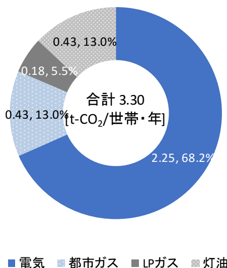
図 1 世帯当たり年間エネルギー種別 CO 2 排出量・構成比（全国）
