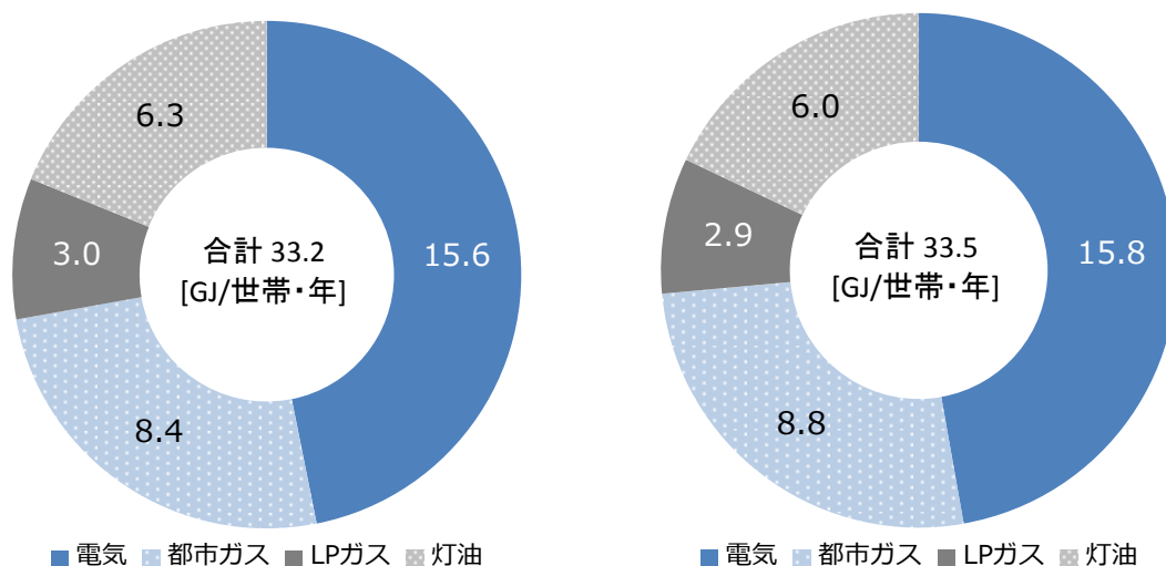
図 2.2.1 世帯当たり年間エネルギー種別消費量（左：平成 29 年度調査／右：全国試験調査）
