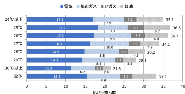
図 14 エアコン (1 台目) の冷房時の設定温度別世帯あたり年間エネルギー消費量
