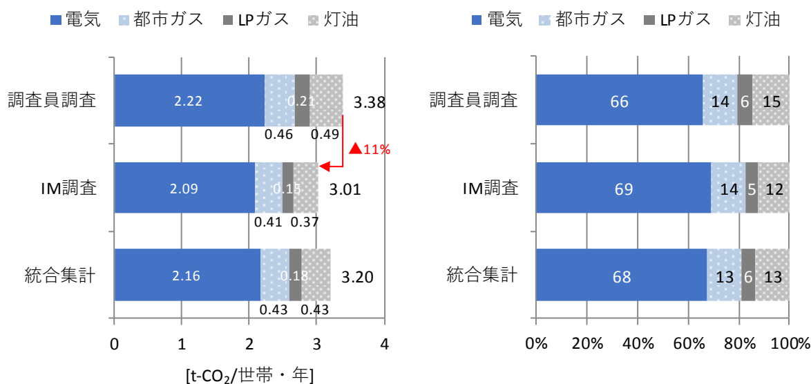
図 2.2.40 調査方式別世帯当たり年間エネルギー種別 CO 2 排出量（H29 調査）
