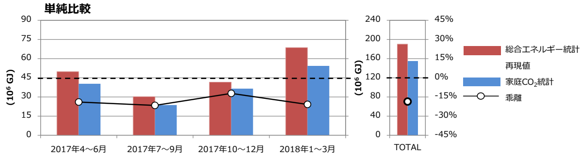
図 2.2.30 総合エネルギー統計試算値と家庭 CO 2 統計の四半期別乖離 (LP ガス) (単純比較)
