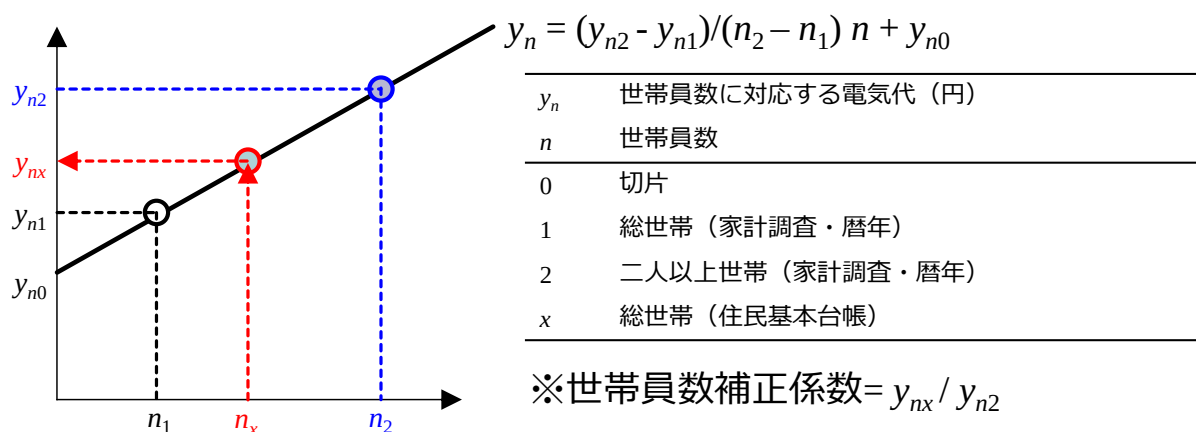
図 2.2.16 電力消費量推計における世帯員数補正の概念図
