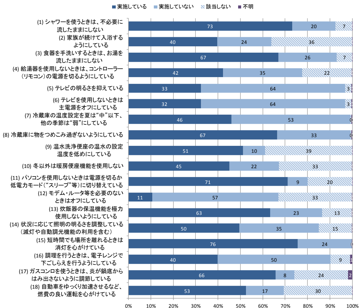
図 2.3.4 省エネルギー行動の実施状況 (H29 年度調査)
