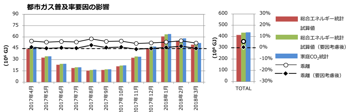
図 2.2.27 総合エネルギー統計試算値と家庭 CO 2 統計の月別乖離（都市ガス） （都市ガス普及率要因の影響）
