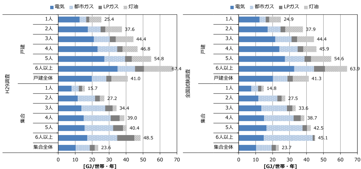
図 2.2.5 建て方別世帯人数別世帯当たり年間エネルギー種別消費量 (左：平成 29 年度調査／右：全国試験調査)
