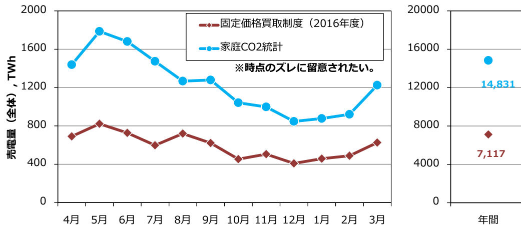
図 4.1.2 固定価格買取制度 (2016 年度) と家庭 CO 2 統計 (2017 年度) の比較 (売電量)
