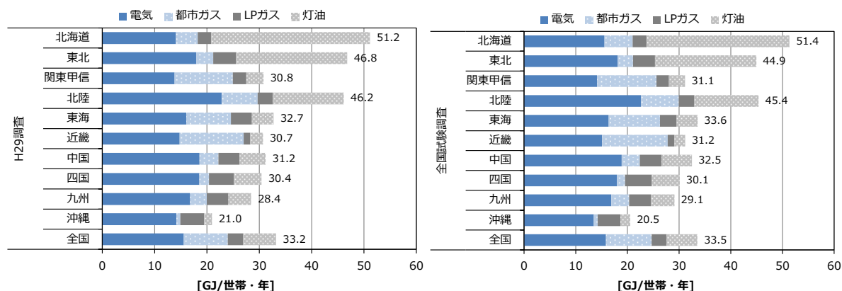
図 2.2.2 地方別世帯当たり年間エネルギー種別消費量
