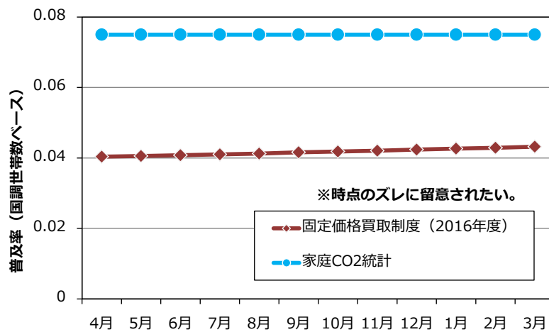
図 4.1.5 固定価格買取制度（2016 年度）と家庭 CO 2 統計（2017 年度）の比較 （普及率（2015 年国勢調査ベース））
