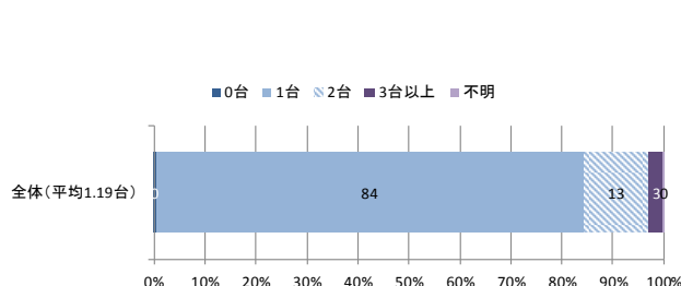
図 11 冷蔵庫の使用台数
