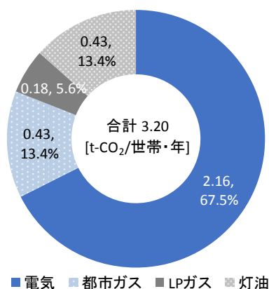
図 1 世帯あたり年間エネルギー種別 CO 2 排出量・構成比（全国）
