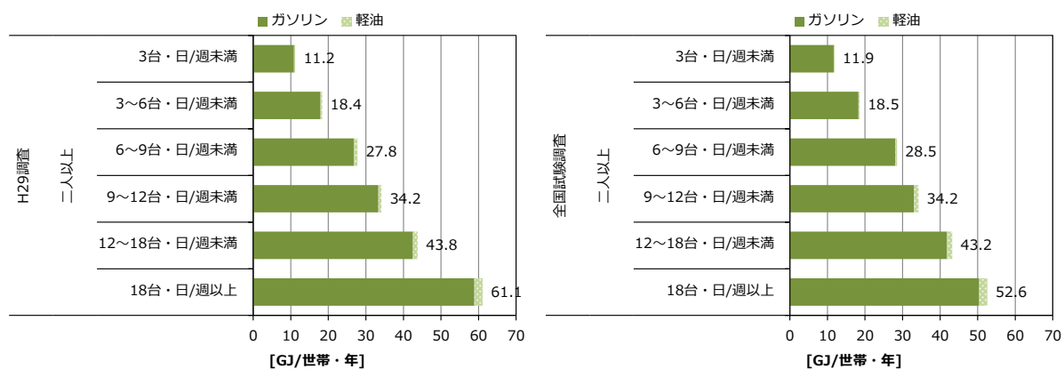
図 2.2.14 自動車（3 台合計）使用頻度別世帯当たり年間自動車燃料種別消費量（二人以上世帯） （左：平成 29 年度調査／右：全国試験調査）
