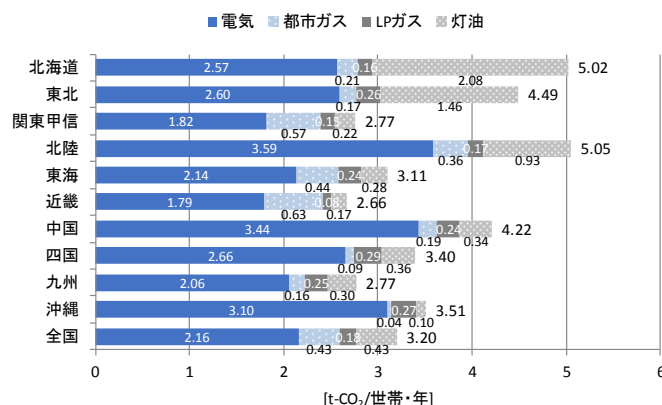
図 2 地方別世帯あたり年間 CO 2 排出量
