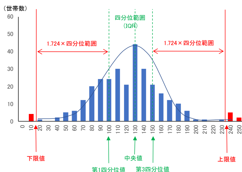
図 5.1.3 中央値及び四分位範囲を用いたレンジチェックの例
