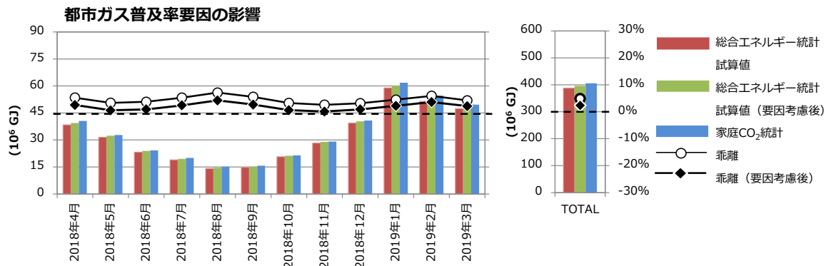
図 2.2.50 総合エネルギー統計試算値と家庭 CO 2 統計の月別乖離（都市ガス） （都市ガス普及率要因の影響）
