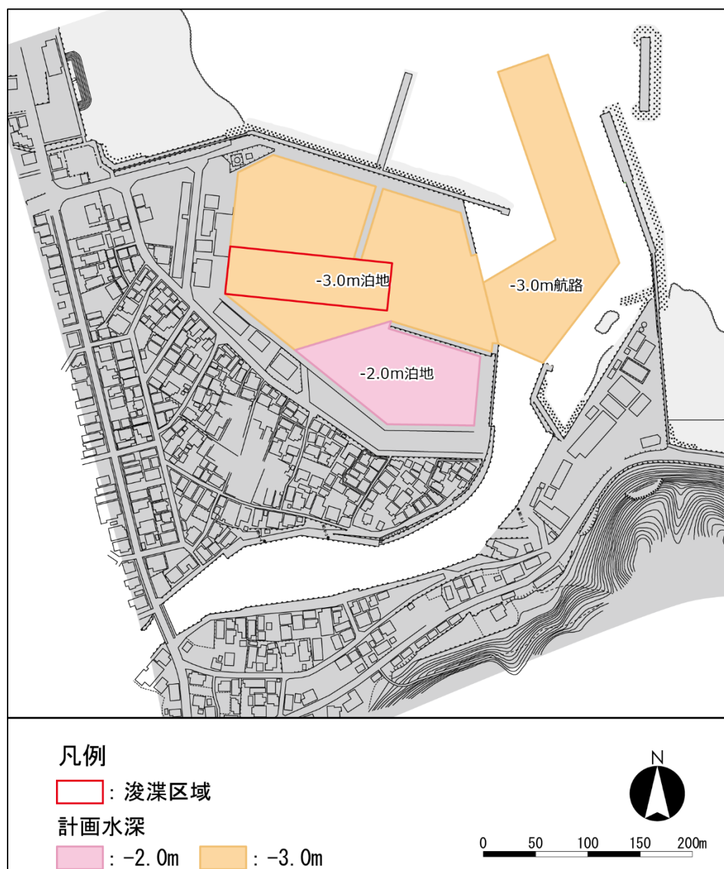
図-2.1 浚渫区域及びその周辺の計画水深
