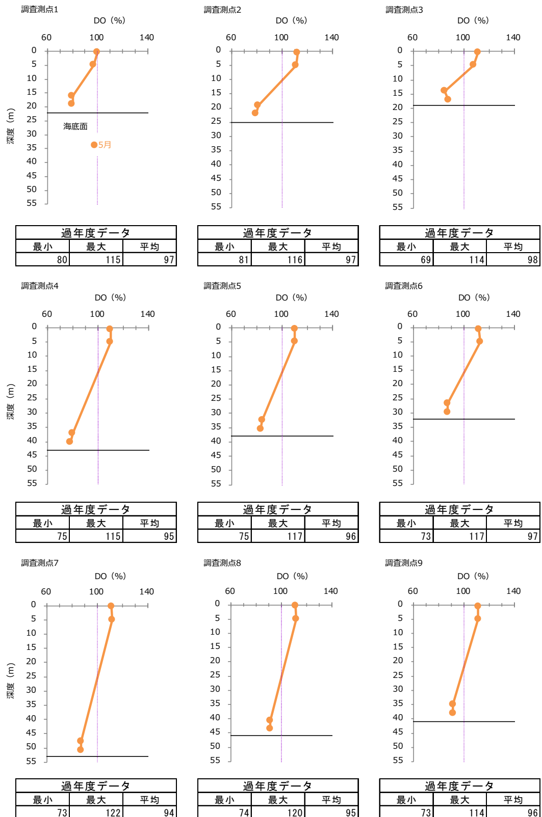
図-16 2024 年度春季 各調査測点における溶存酸素（DO）飽和度の鉛直プロファイル
