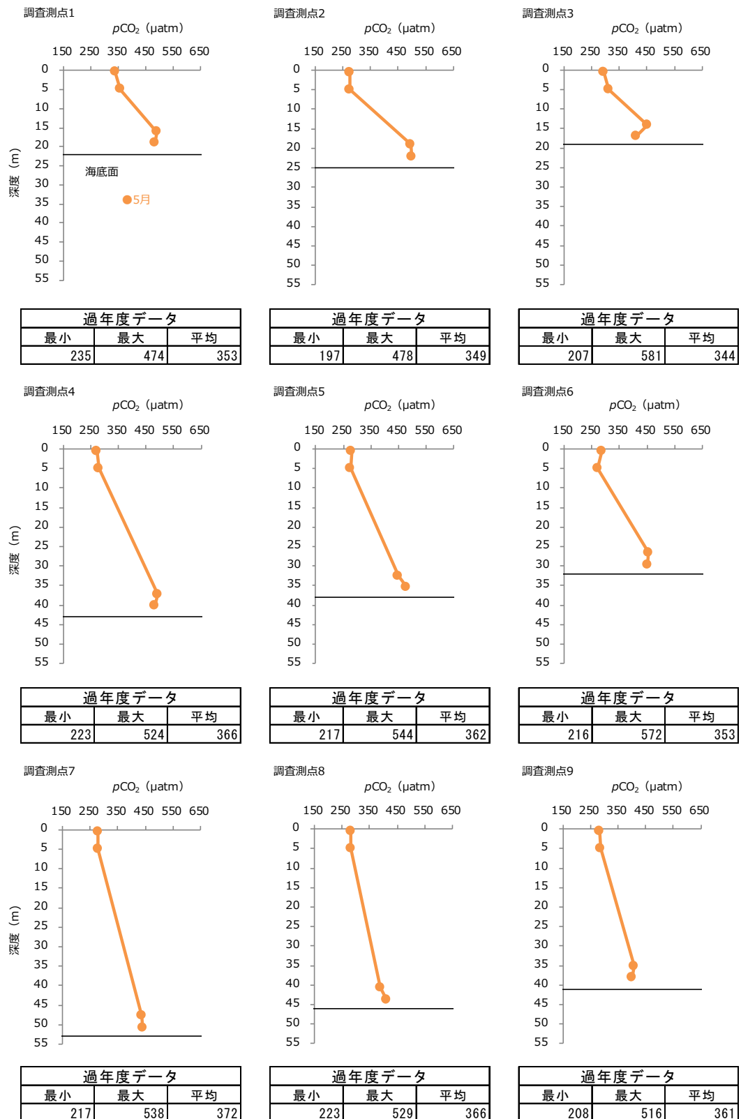
図-14 2024 年度春季 各調査測点における二酸化炭素分圧 ( p\text{CO}_2 ) の鉛直プロファイル
