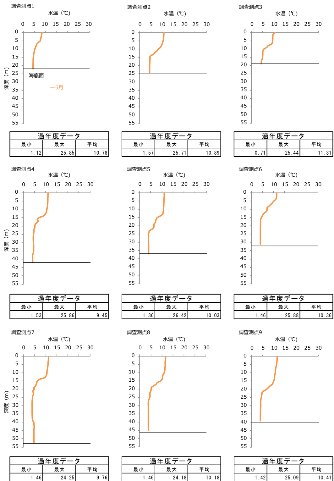
図-2 2024 年度春季 各調査測点における水温の鉛直プロファイル
