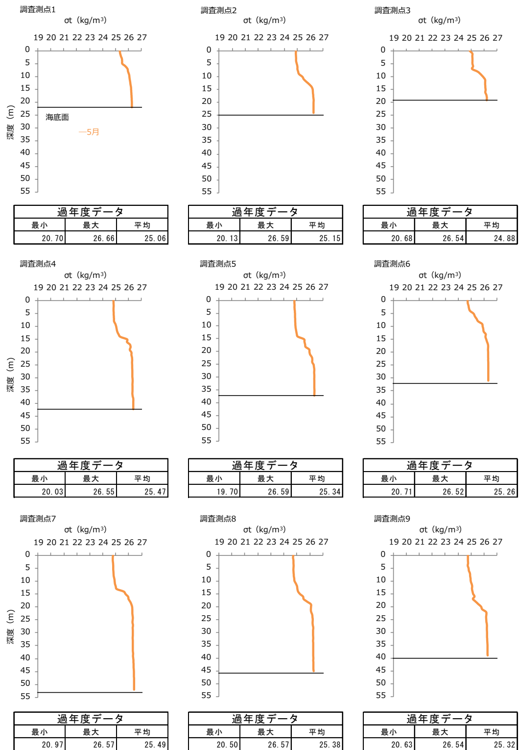
図-6 2024 年度春季 各調査測点における海水密度（ \sigma_t ）の鉛直プロファイル
