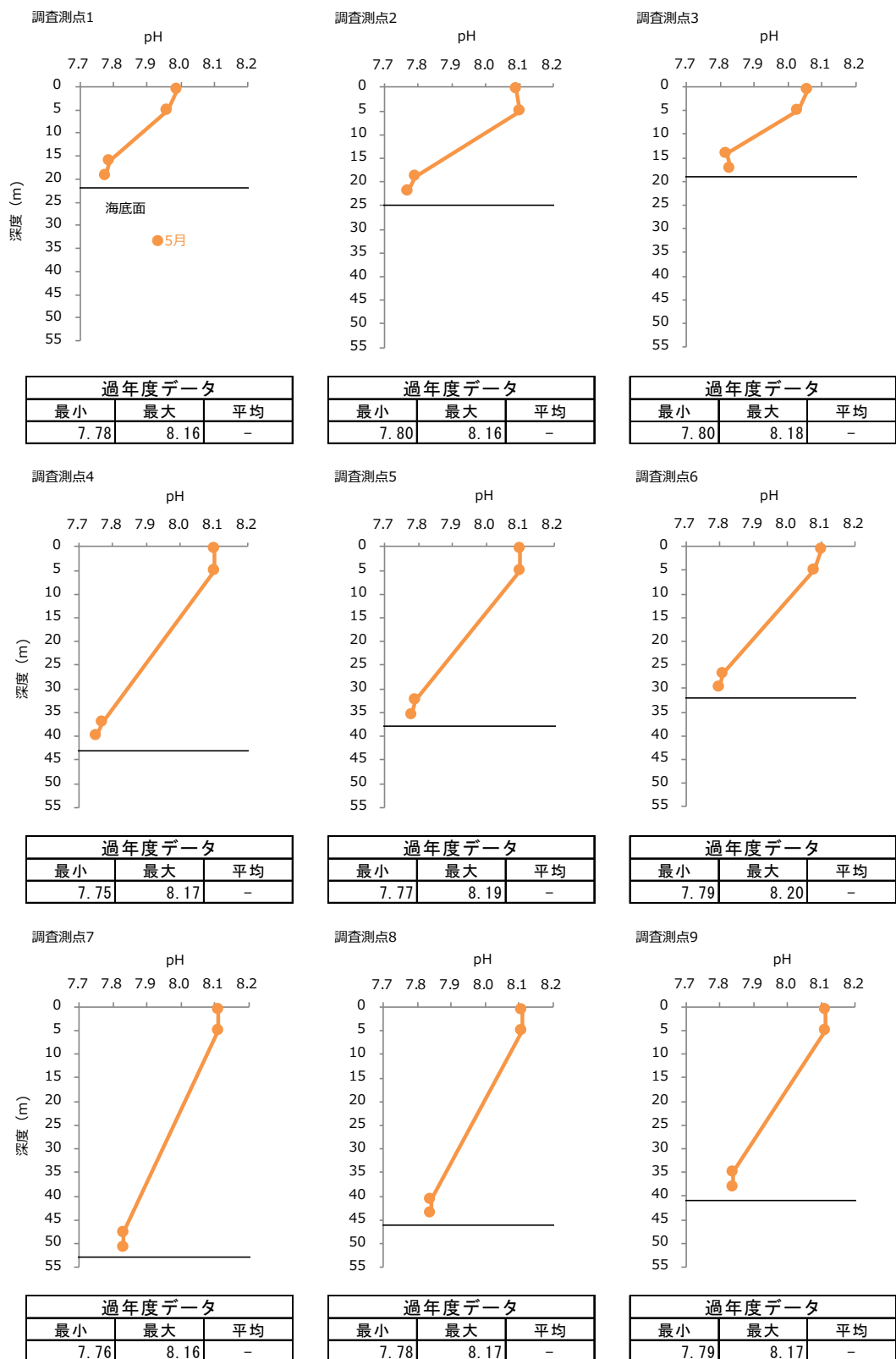
図-12 2024 年度春季 各調査測点における pH の鉛直プロファイル
