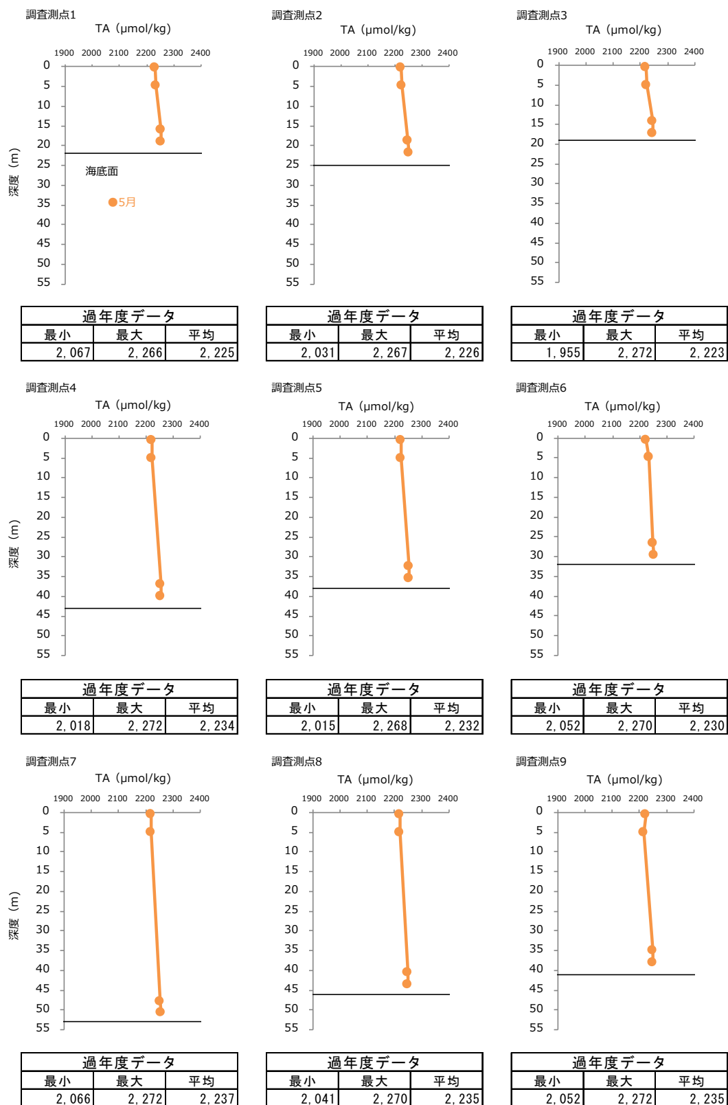
図-8 2024 年度春季 各調査測点におけるアルカリ度（TA）の鉛直プロファイル
