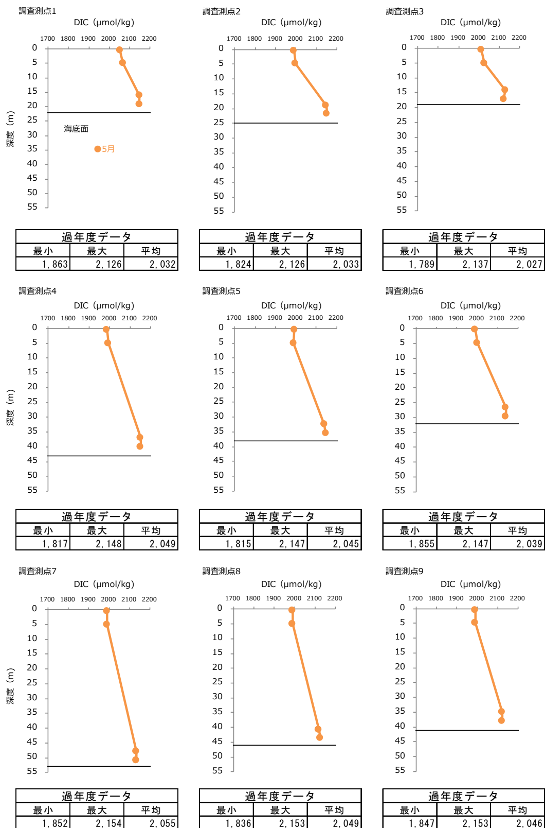
図-10 2024 年度春季 各調査測点における全炭酸（DIC）濃度の鉛直プロファイル
