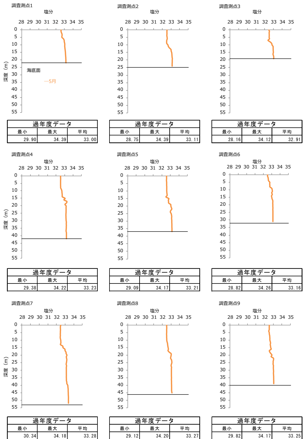
図-4 2024 年度春季 各調査測点における塩分の鉛直プロファイル
