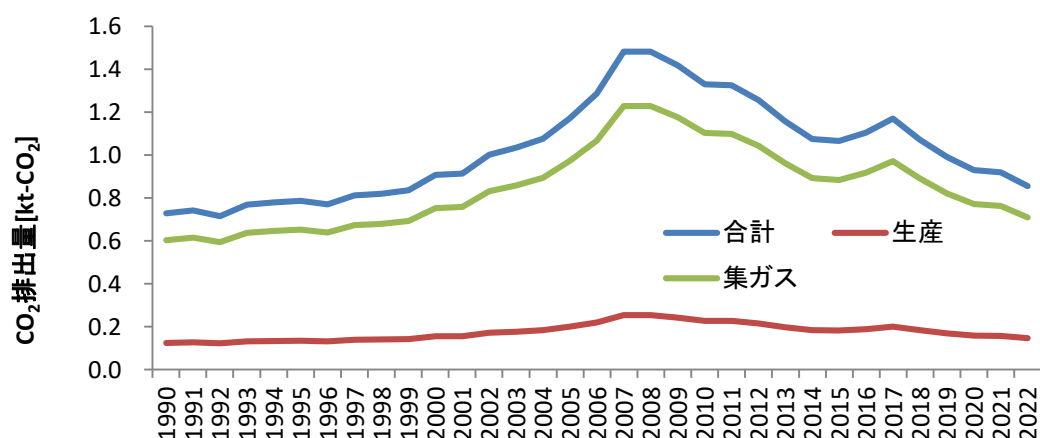
図 1 天然ガス生産時からの CO 2 排出量の推移
