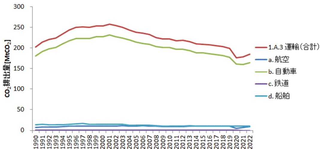
図 1 「1.A.3. 運輸」からの CO 2 排出量の推移
