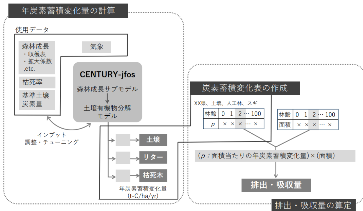
図 4 CENTURY-jfos モデルの概要
