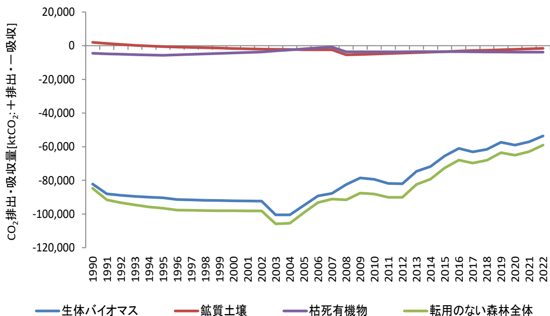
図 3 転用のない森林における CO 2 排出・吸収量の推移
