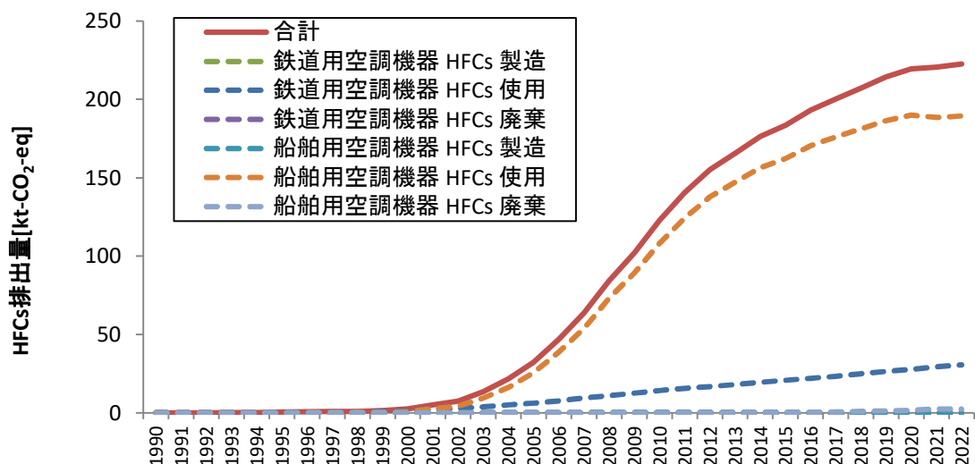
図 2 「2.F.1.- 輸送機器用空調機器の製造、使用及び廃棄（鉄道・船舶）」からの HFCs 排出量の推移
