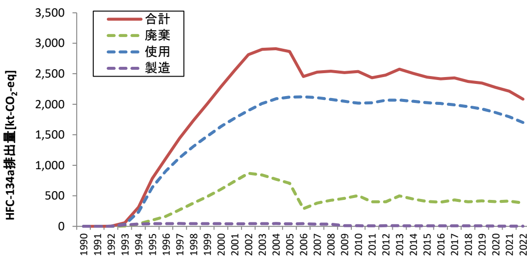
図 1 「2.F.1.- 輸送機器用空調機器の製造、使用及び廃棄（カーエアコン）」からの HFC-134a 排出量の推移
