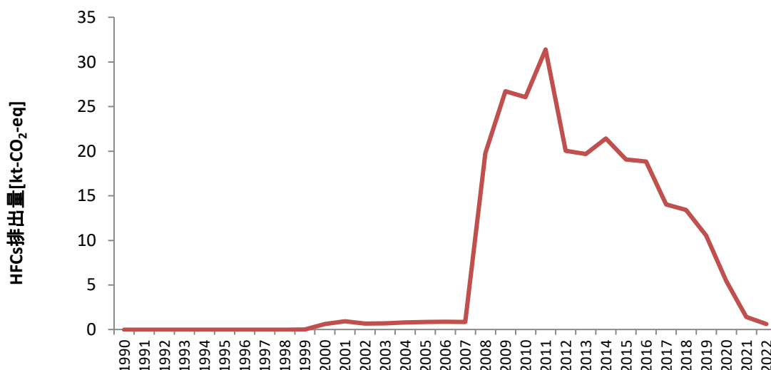
図 1 「2.F.1.- 自動販売機の製造、使用及び廃棄」からの HFCs 排出量の推移
