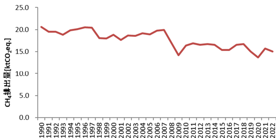
図 2 鋼製造（電気炉）からの CH 4 排出量の推移
