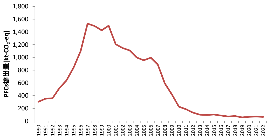
図 2 「2.B.9.- 製造時の漏出」からの PFCs 排出量の推移
