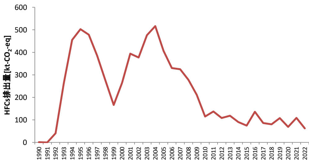
図 1 「2.B.9.- 製造時の漏出」からの HFCs 排出量の推移
