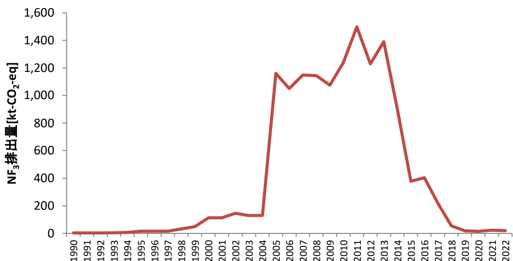
図 4 「2.B.9.- 製造時の漏出」からの NF 3 排出量の推移
