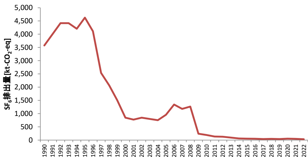
図 3 「2.B.9.- 製造時の漏出」からの SF 6 排出量の推移
