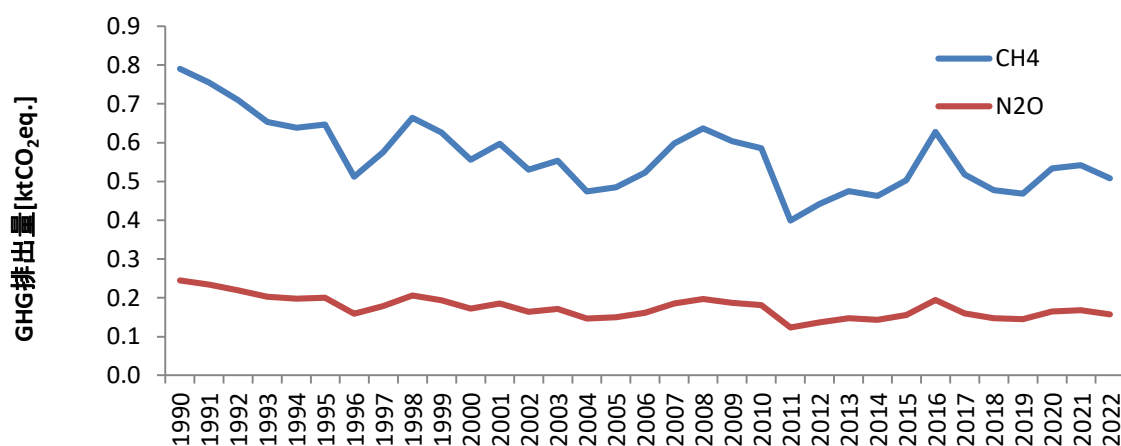
図 1 さとうきびの残さの野焼きからの CH 4 及び N 2 O 排出量の推移
