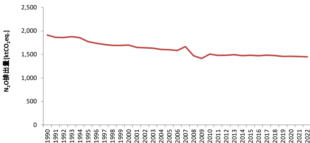
図 1 間接排出（窒素溶脱・流出）からの N 2 O 排出量の推移
