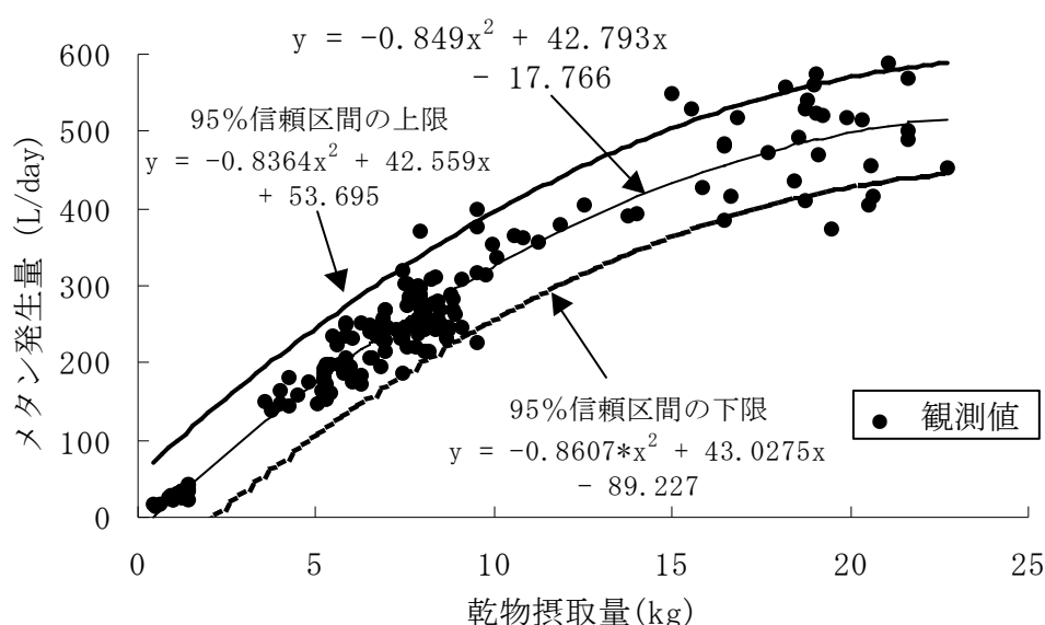
図 2 柴田（1993）における観測値と CH 4 発生量算出式
