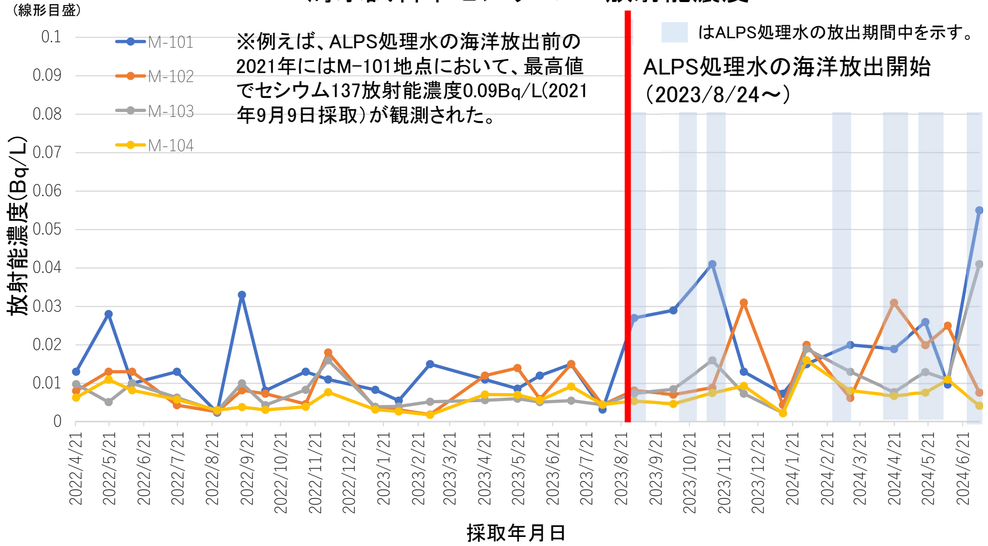
海水試料中セシウム137放射能濃度
