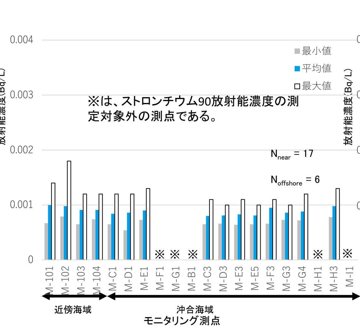
(線形目盛) 海水試料中ストロンチウム90放射能濃度 (線形目盛) 放出前 採取期間: 2022年4月21日～2023年8月4日
