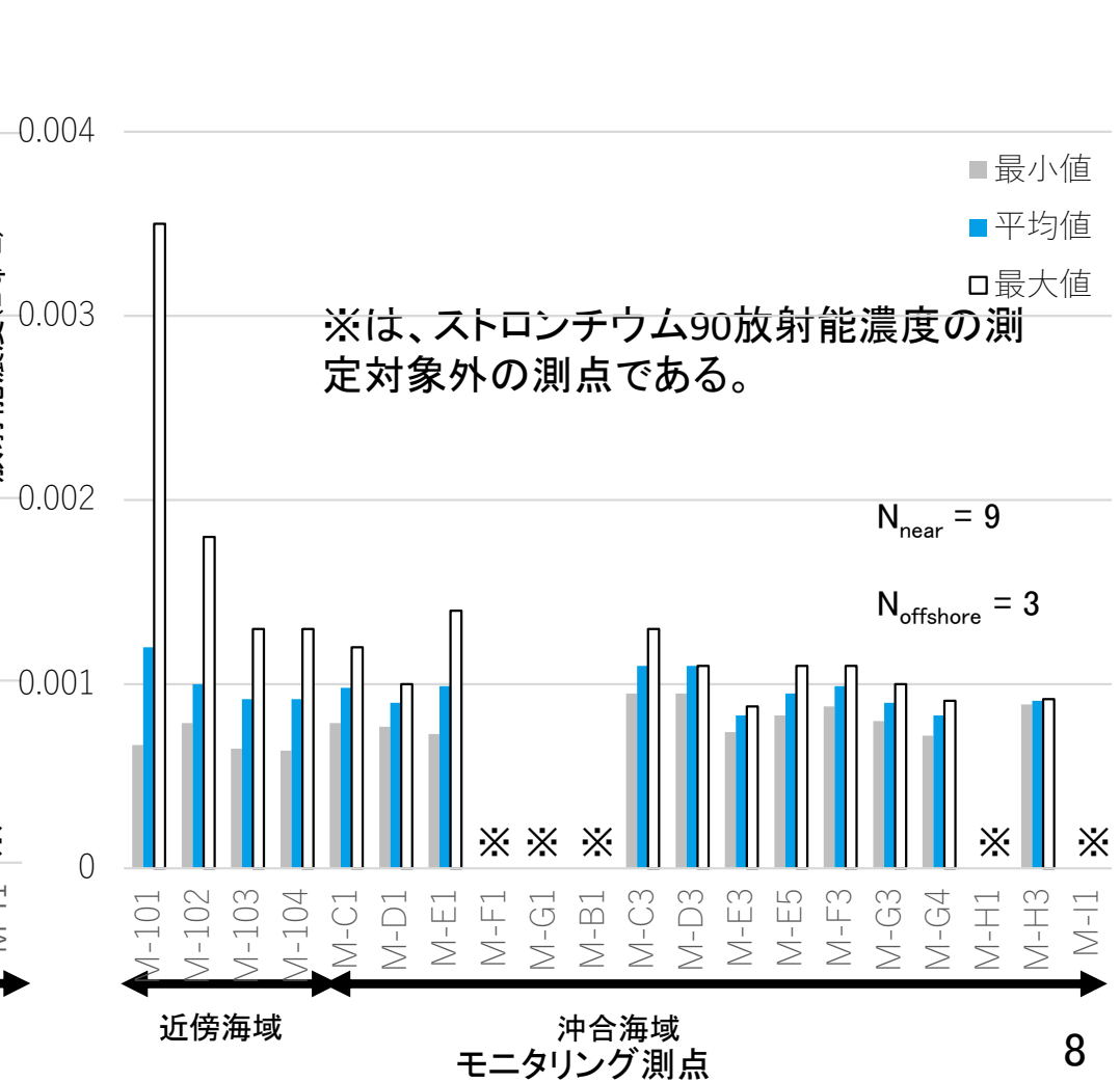
(線形目盛) 海水試料中ストロンチウム90放射能濃度 放出開始後 採取期間: 2023年9月1日～2024年5月26日
