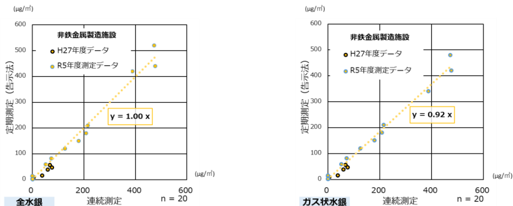
図 10 告示法と連続測定法の相関図（石炭火力発電所）（左：全水銀、右：ガス状水銀）
