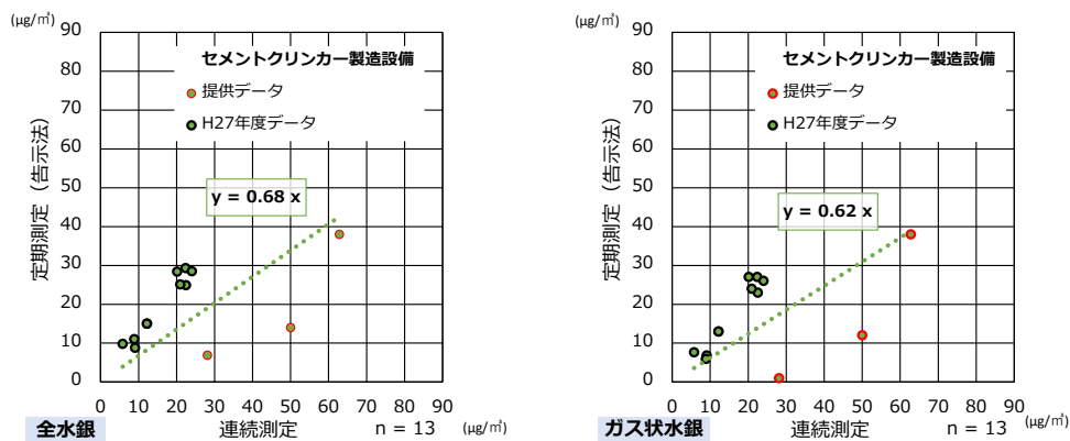
図 11 告示法と連続測定法の相関図（非鉄金属製造施設）（左：全水銀、右：ガス状水銀）
