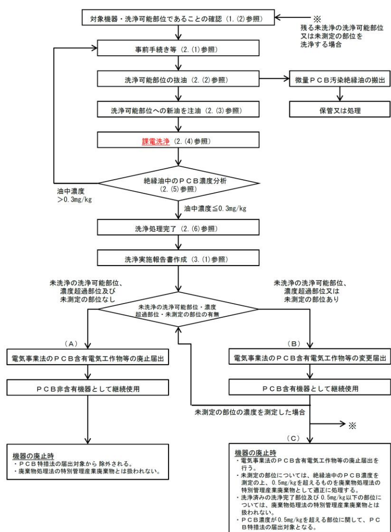
図1 課電洗浄フロー図
