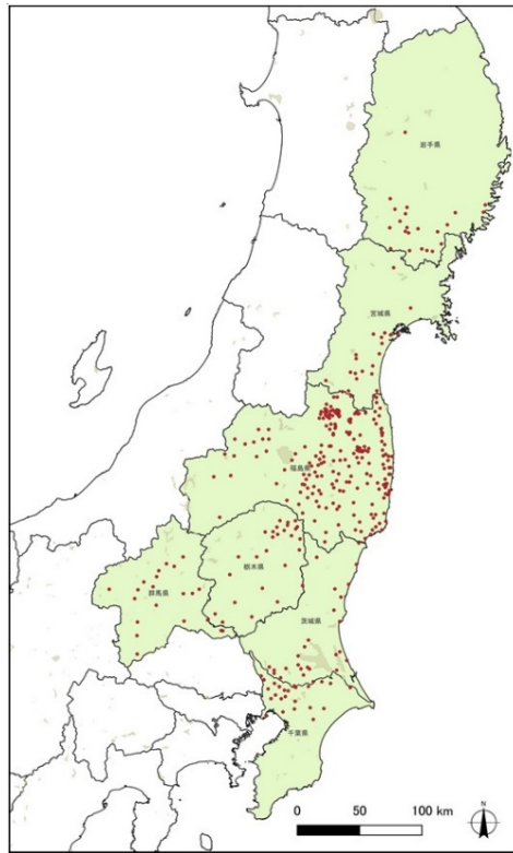
②地下水
