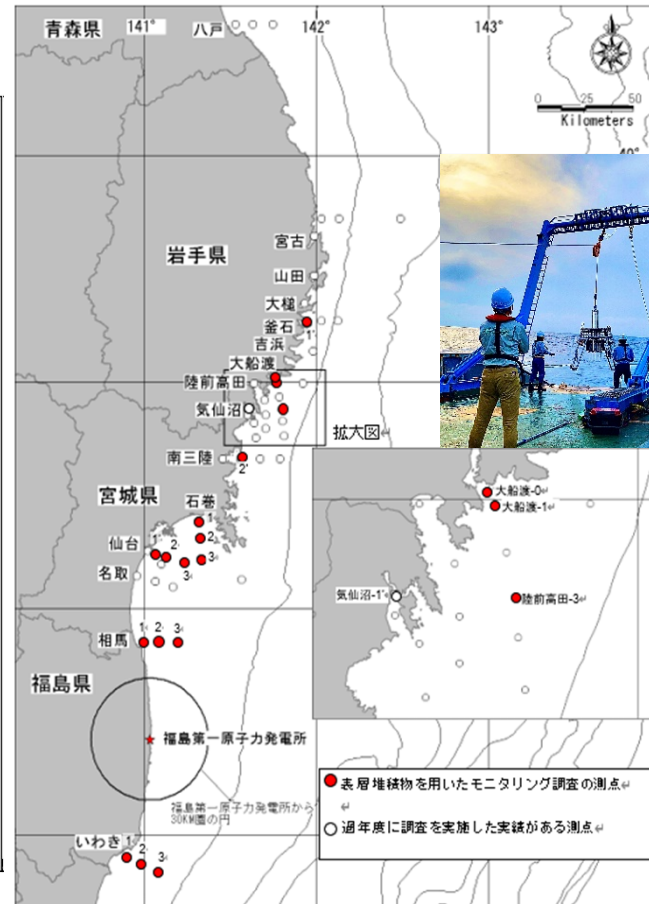
③海洋
