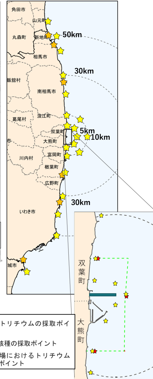
④ALPS処理水
