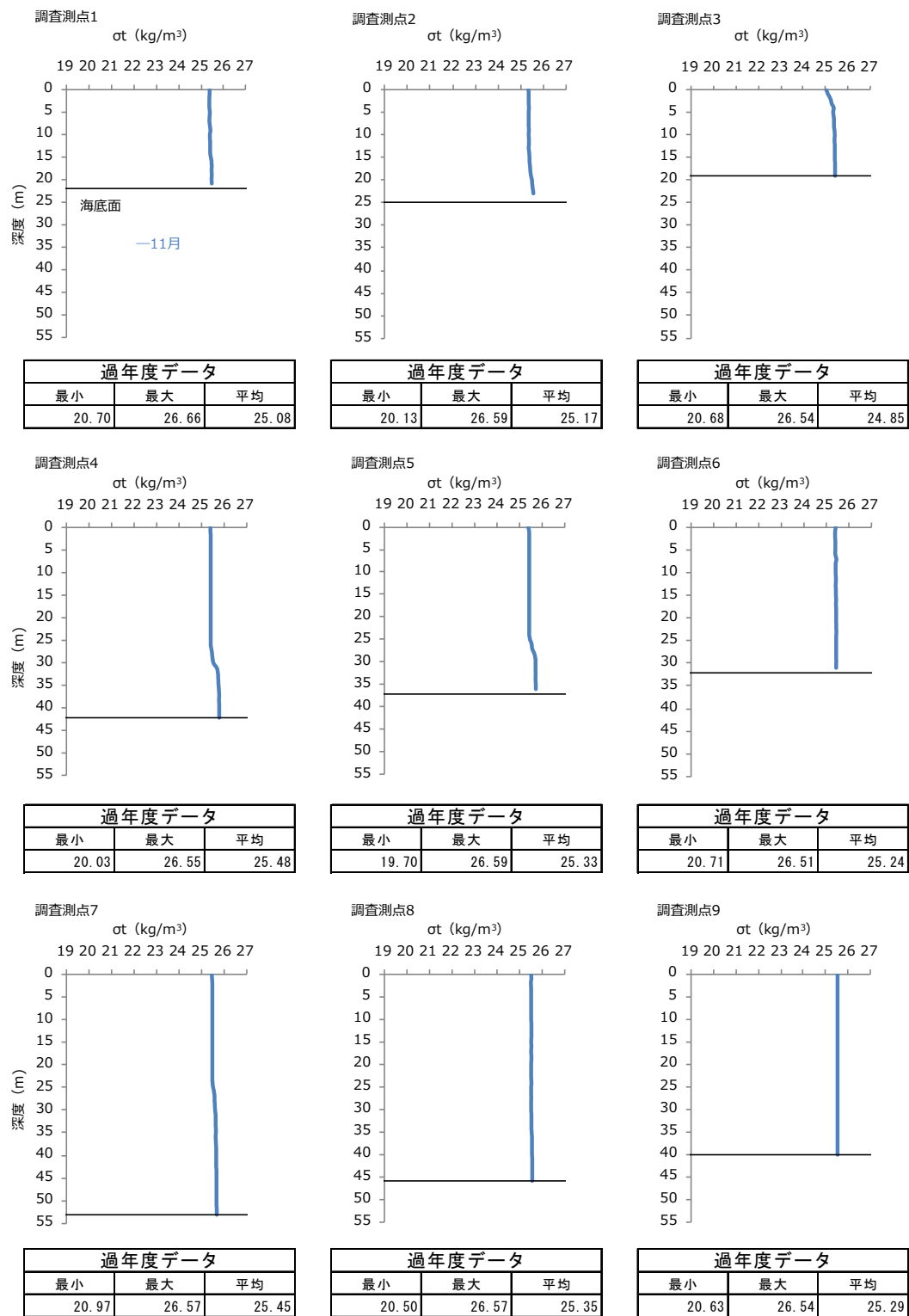
図-6 2022 年度秋季 各調査測点における海水密度（ \sigma_t ）の鉛直プロファイル
