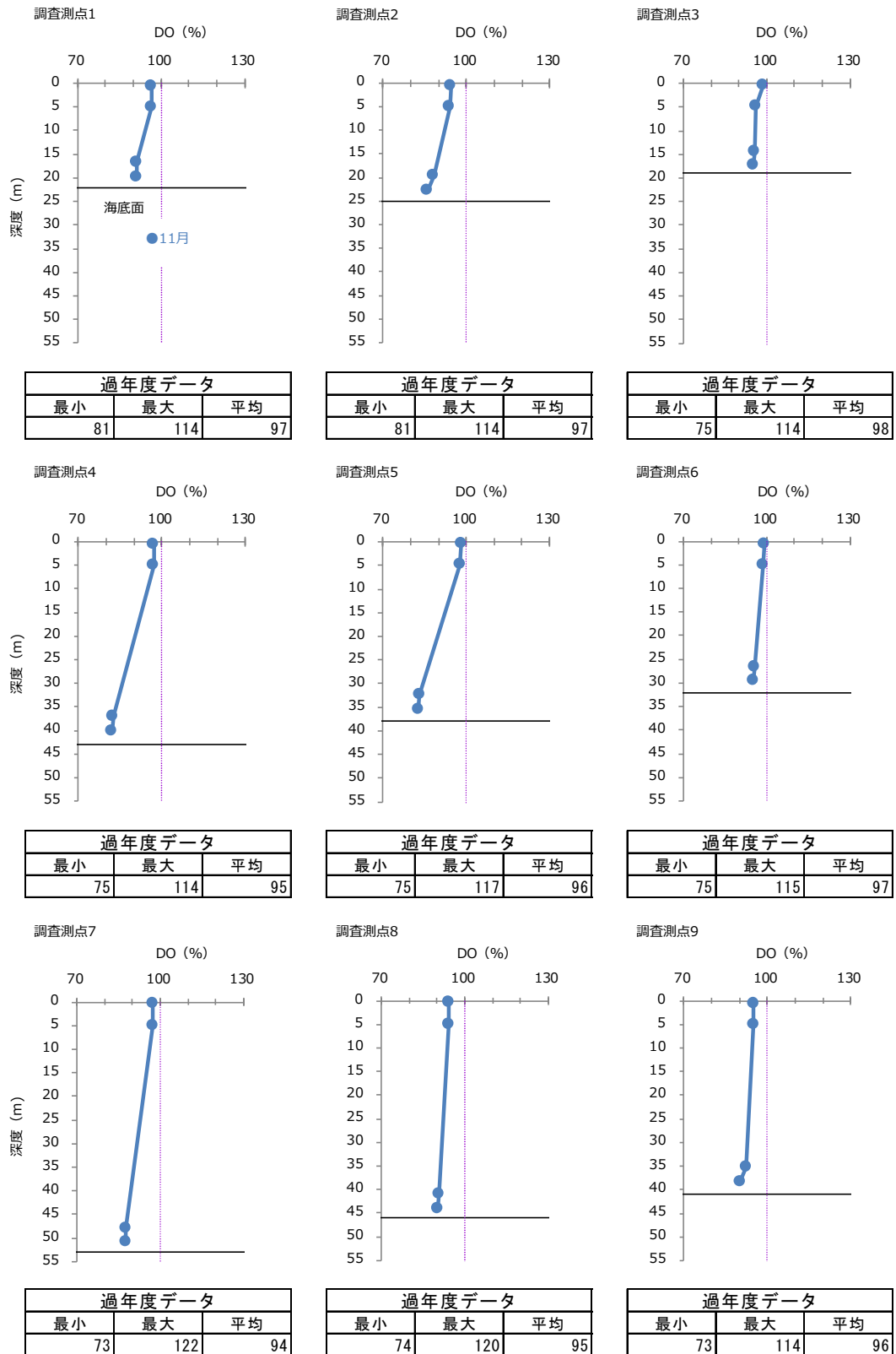
図-16 2022 年度秋季 各調査測点における溶存酸素 (DO) 飽和度の鉛直プロファイル
