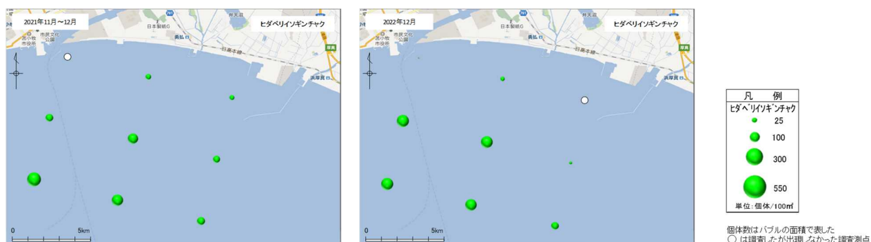
図-23 ROV 調査による目視観察結果 ヒダベリイソギンチャクの出現状況 (個体/100m²)
