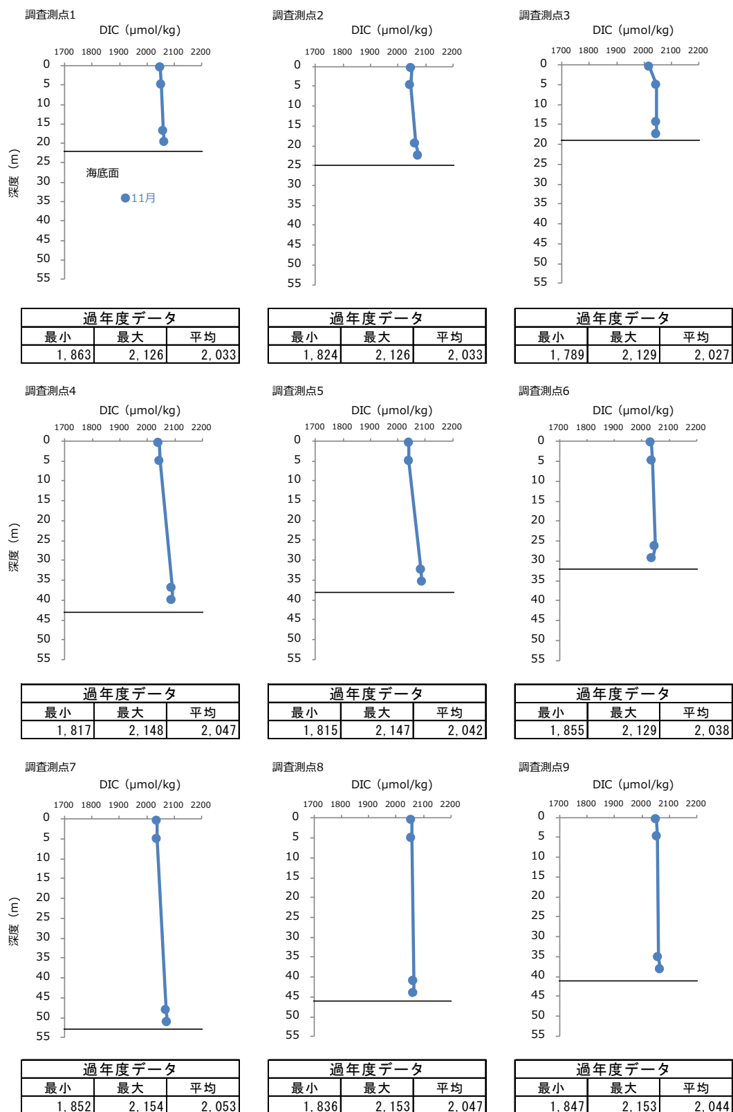
図-10 2022 年度秋季 各調査測点における全炭酸（DIC）濃度の鉛直プロファイル
