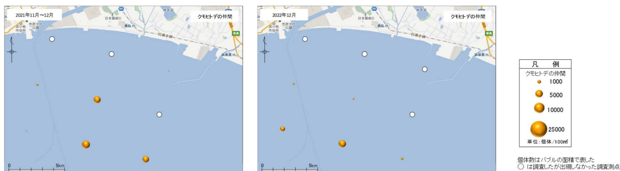
図-22 ROV 調査による目視観察結果 クモヒトデ綱の出現状況 (個体/100m²)
