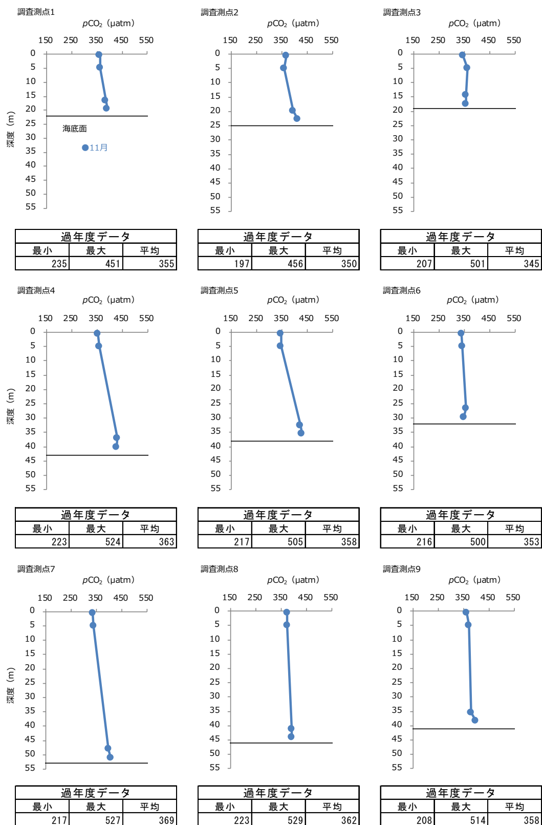
図-14 2022 年度秋季 各調査測点における二酸化炭素分圧 ( p\text{CO}_2 ) の鉛直プロファイル
