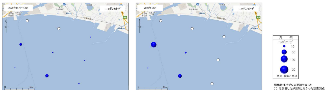
図-21 ROV 調査による目視観察結果 ニッポンヒトデの出現状況 (個体/100m²)
