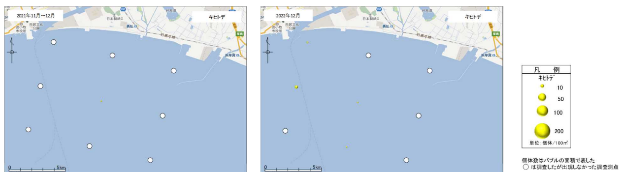
図-20 ROV 調査による目視観察結果 キヒトデの出現状況 (個体/100m²)
