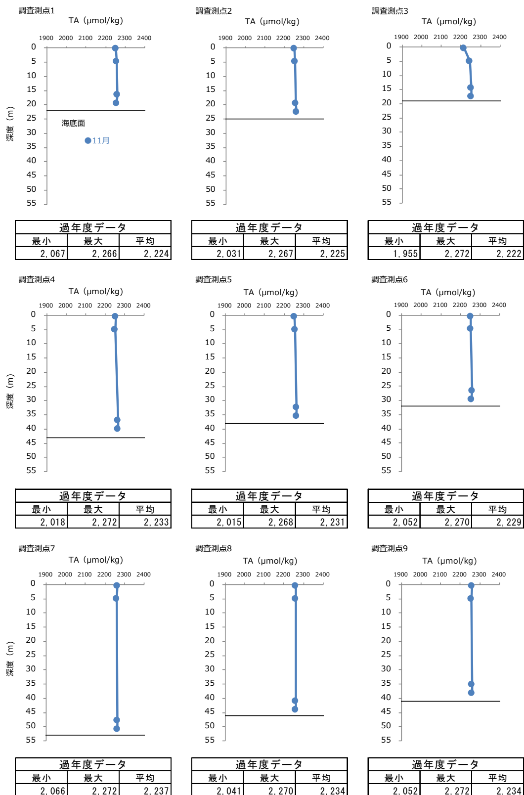
図-8 2022 年度秋季 各調査測点におけるアルカリ度 (TA) の鉛直プロファイル
