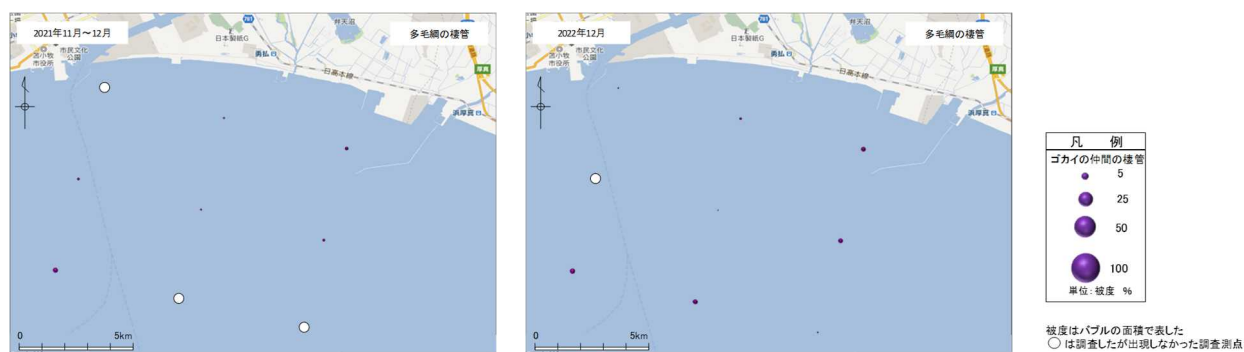
図-24 ROV 調査による目視観察結果 多毛網の棲管の出現状況（被度 %）
