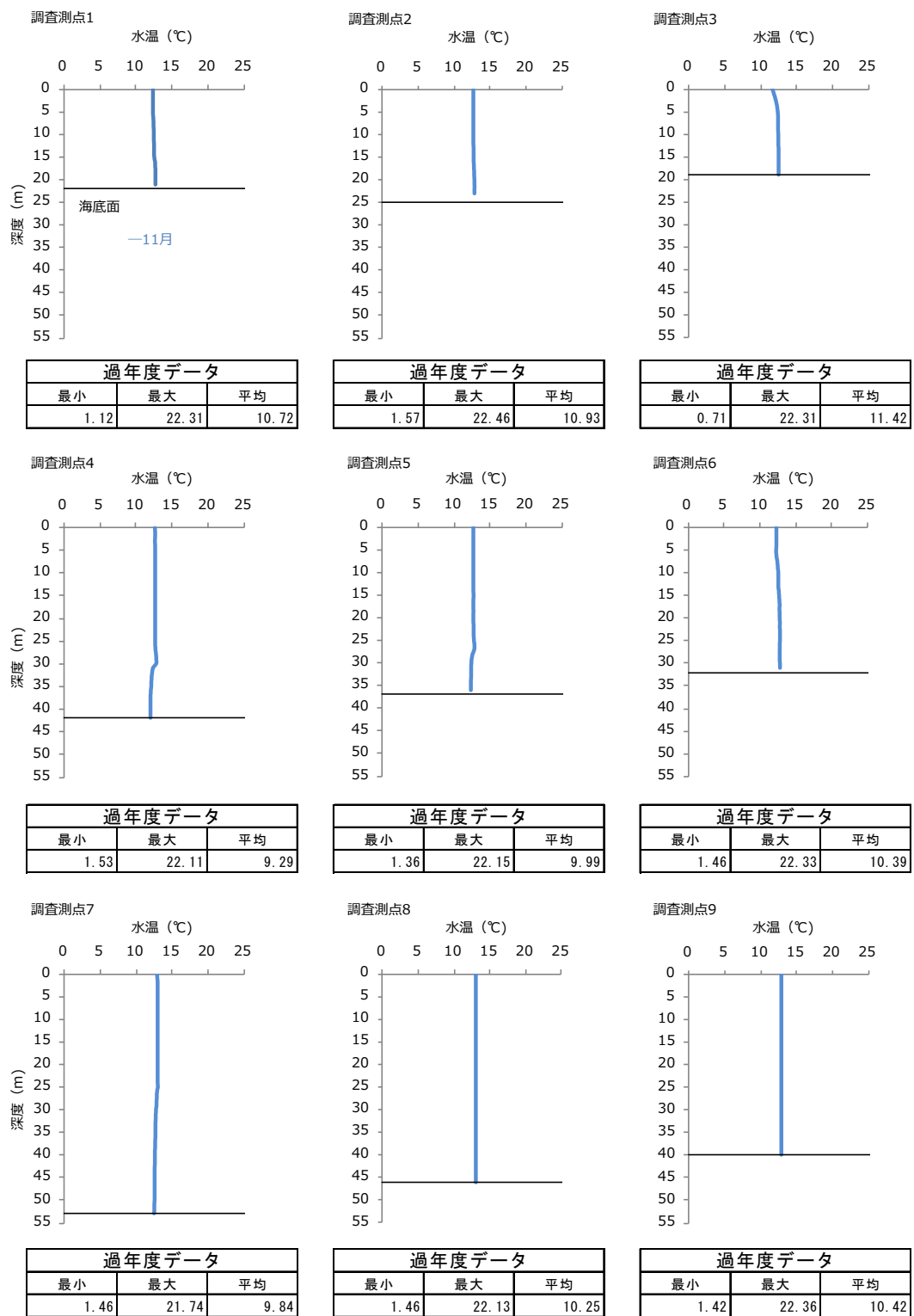
図-2 2022 年度秋季 各調査測点における水温の鉛直プロファイル
