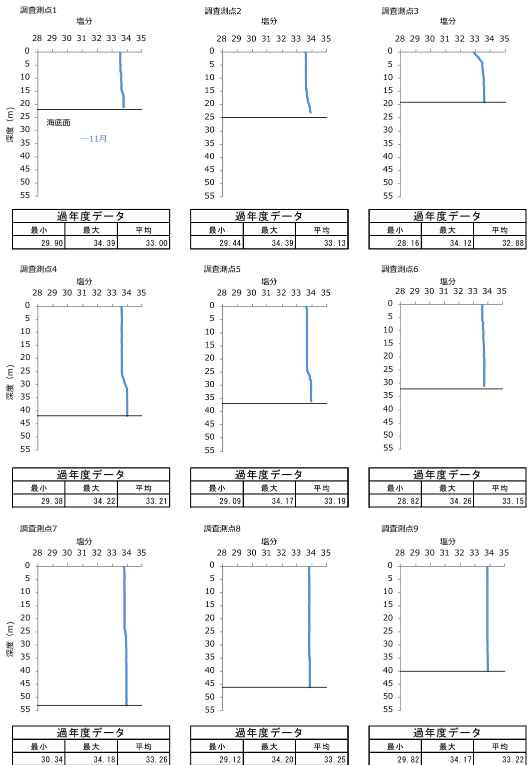
図-4 2022 年度秋季 各調査測点における塩分の鉛直プロファイル
