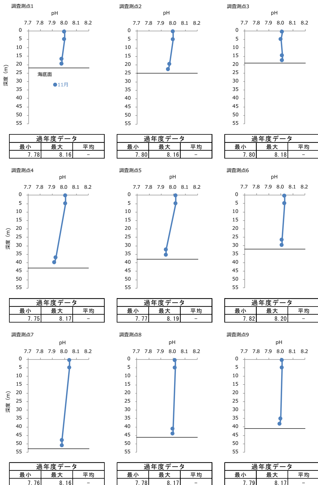
図-12 2022 年度秋季 各調査測点における pH の鉛直プロファイル
