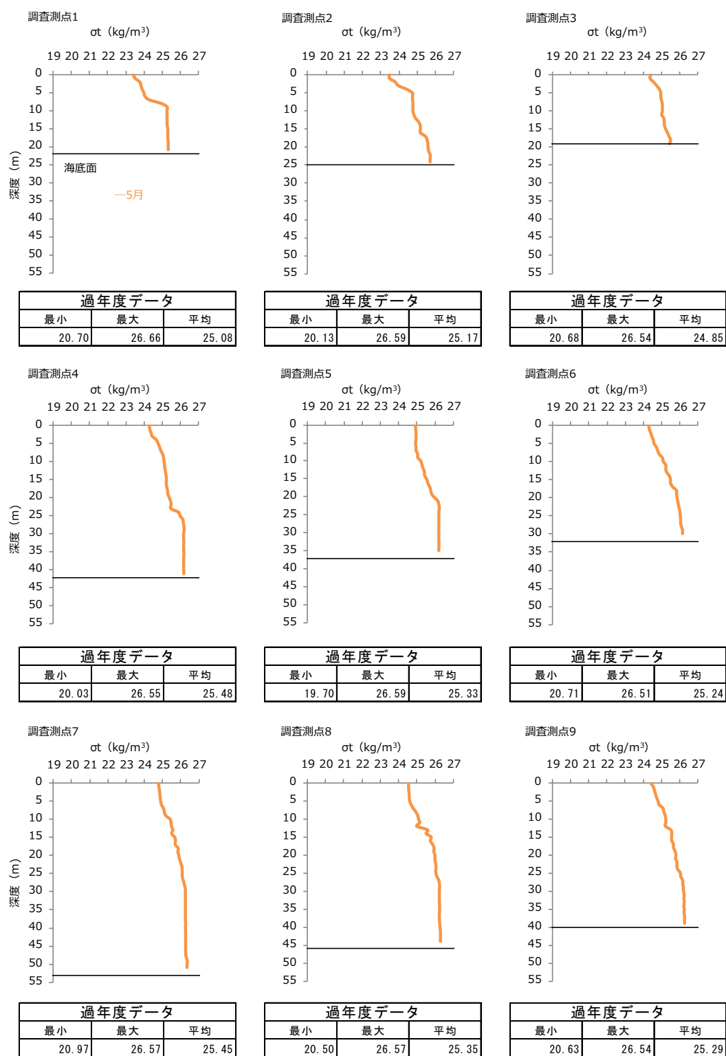
図-6 2022 年度春季 各調査測点における海水密度（ \sigma_t ）の鉛直プロファイル
