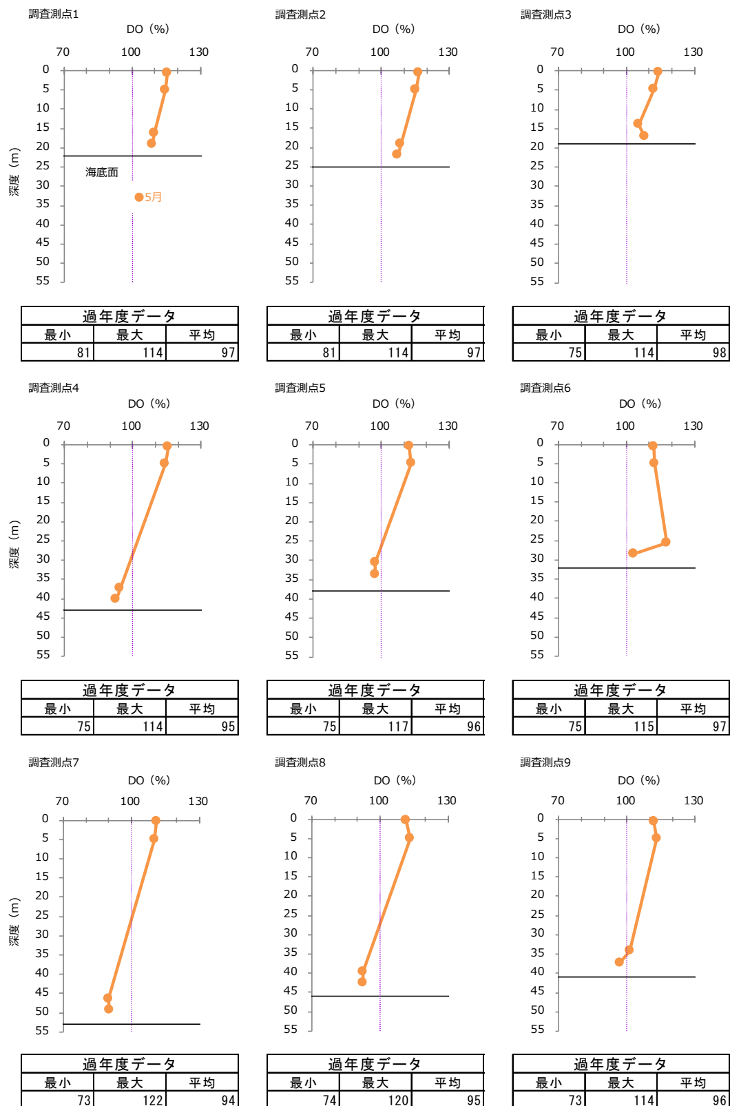
図-16 2022 年度春季 各調査測点における溶存酸素（DO）飽和度の鉛直プロファイル
