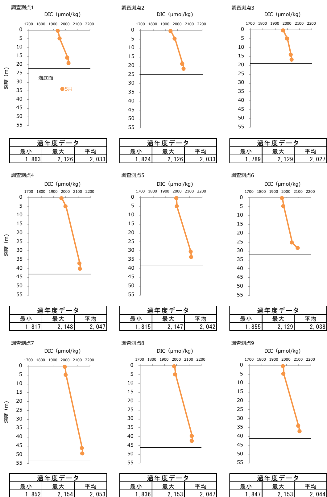
図-10 2022 年度春季 各調査測点における全炭酸（DIC）濃度の鉛直プロファイル
