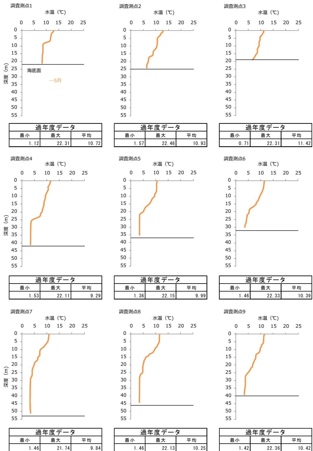
図-2 2022 年度春季 各調査測点における水温の鉛直プロファイル
