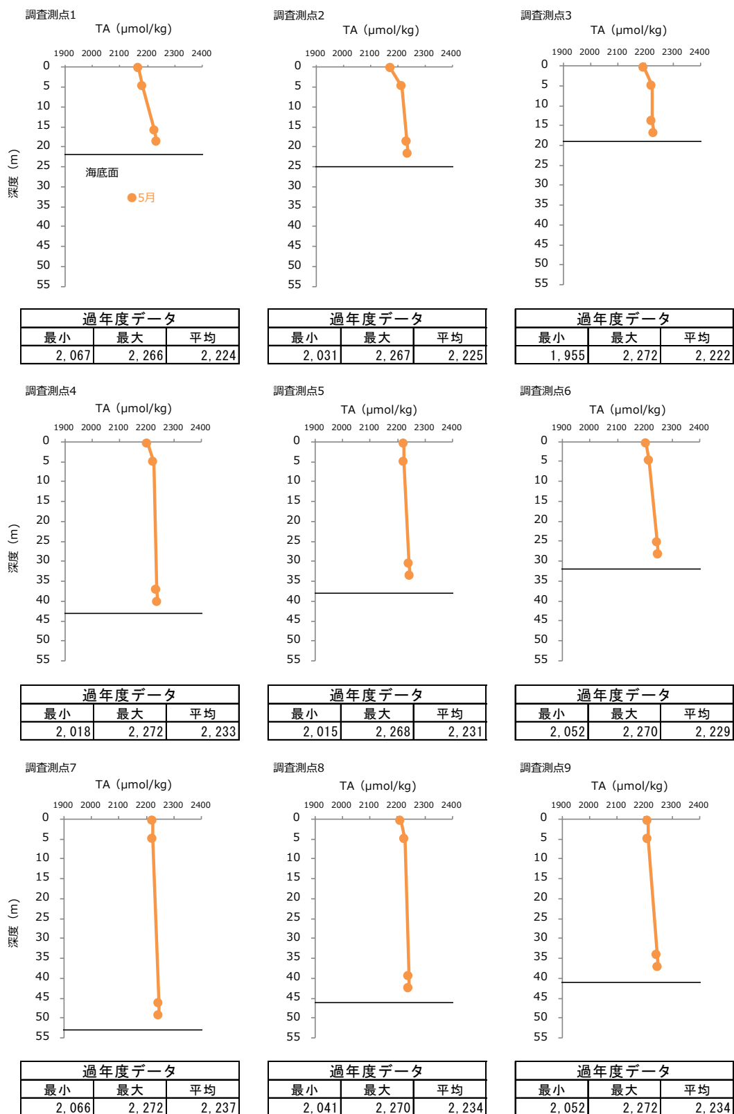
図-8 2022 年度春季 各調査測点におけるアルカリ度 (TA) の鉛直プロファイル
