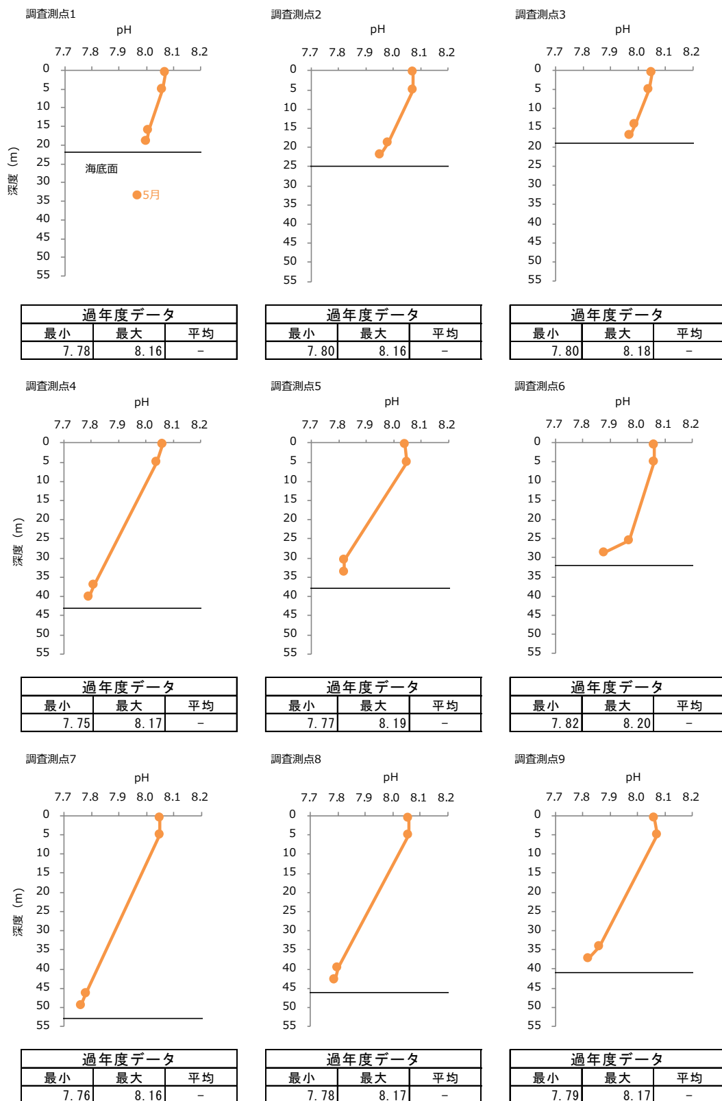
図-12 2022 年度春季 各調査測点における pH の鉛直プロファイル
