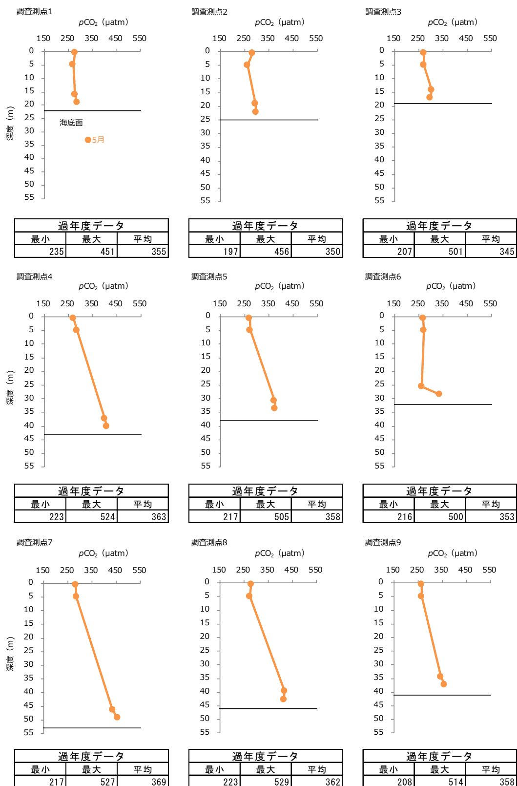
図-14 2022 年度春季 各調査測点における二酸化炭素分圧 ( p\text{CO}_2 ) の鉛直プロファイル
