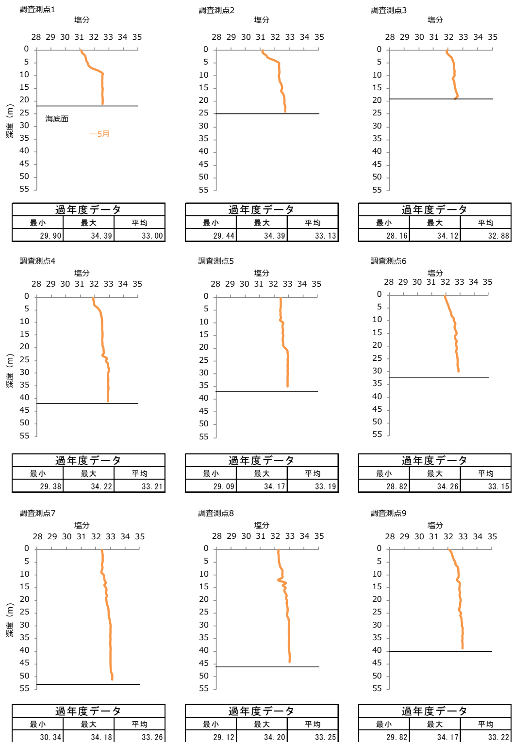
図-4 2022 年度春季 各調査測点における塩分の鉛直プロファイル
