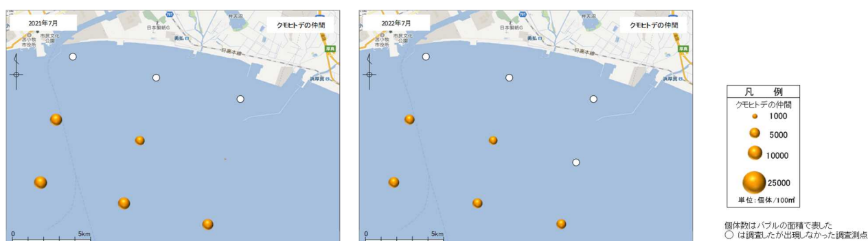
図-22 ROV 調査による目視観察結果 クモヒトデ網の出現状況 (個体/100m 2 )
