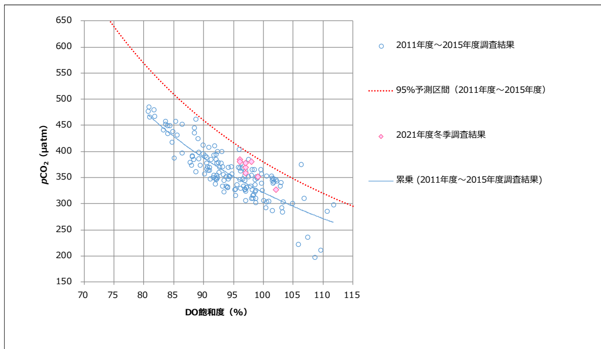
図 5 p\text{CO}_2 と DO 飽和度との関係
