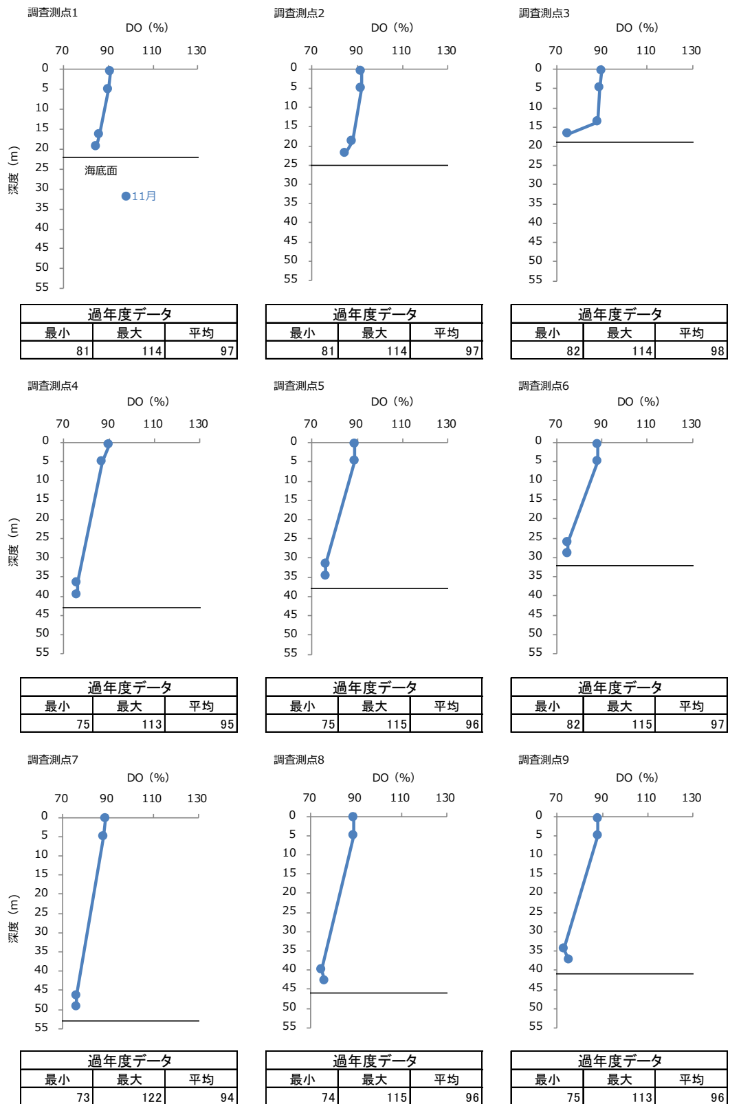
図-16 2021 年度秋季 各調査測点における溶存酸素 (DO) 飽和度の鉛直プロファイル
