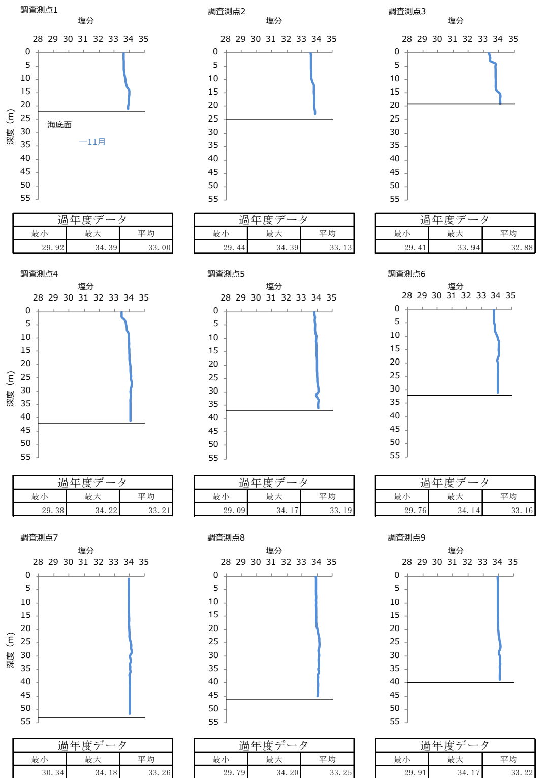
図-4 2021 年度秋季 各調査測点における塩分の鉛直プロファイル
