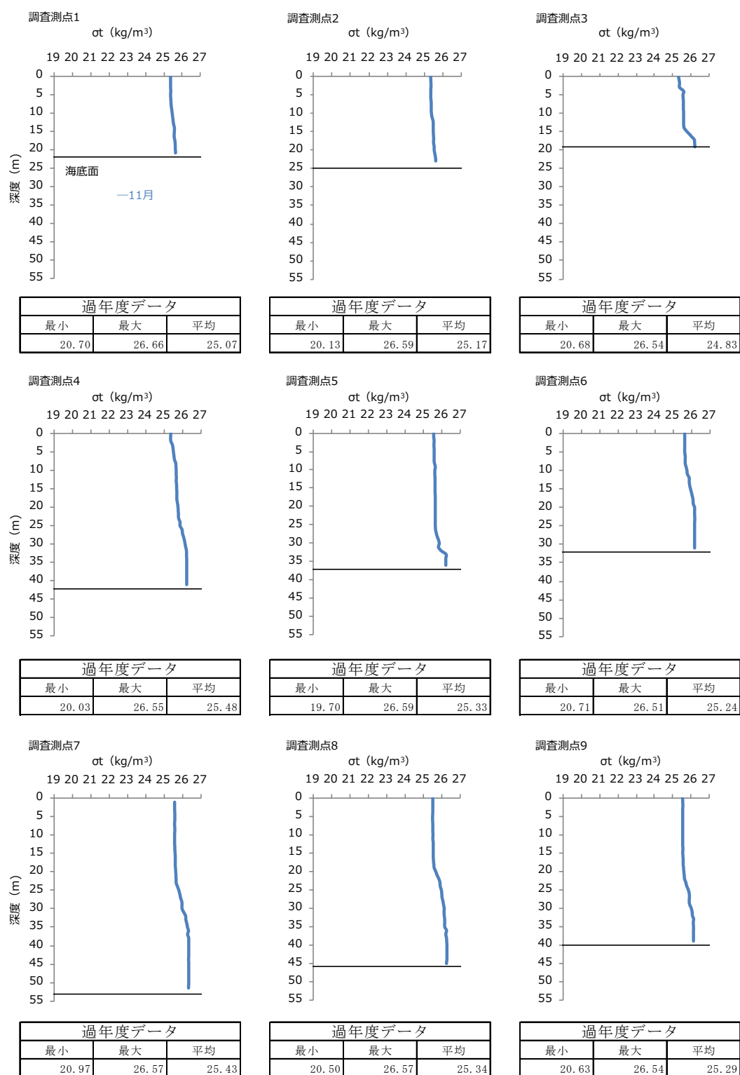
図-6 2021 年度秋季 各調査測点における海水密度 ( \sigma_t ) の鉛直プロファイル
