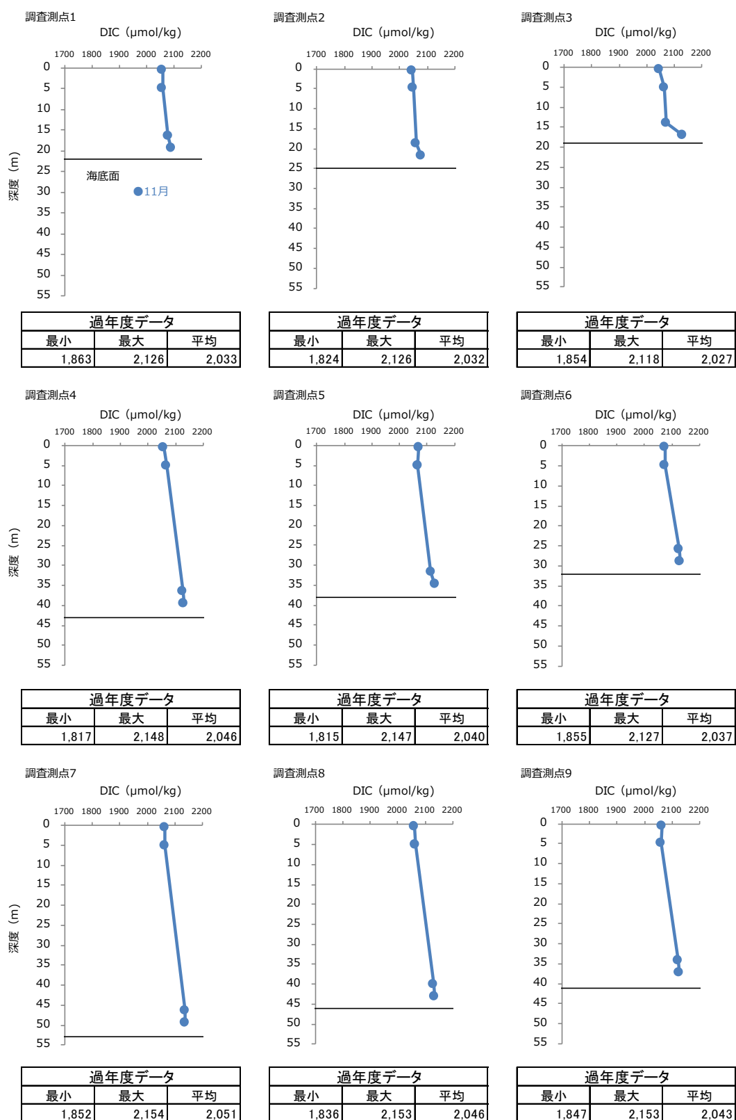
図-10 2021 年度秋季 各調査測点における全炭酸（DIC）濃度の鉛直プロファイル
