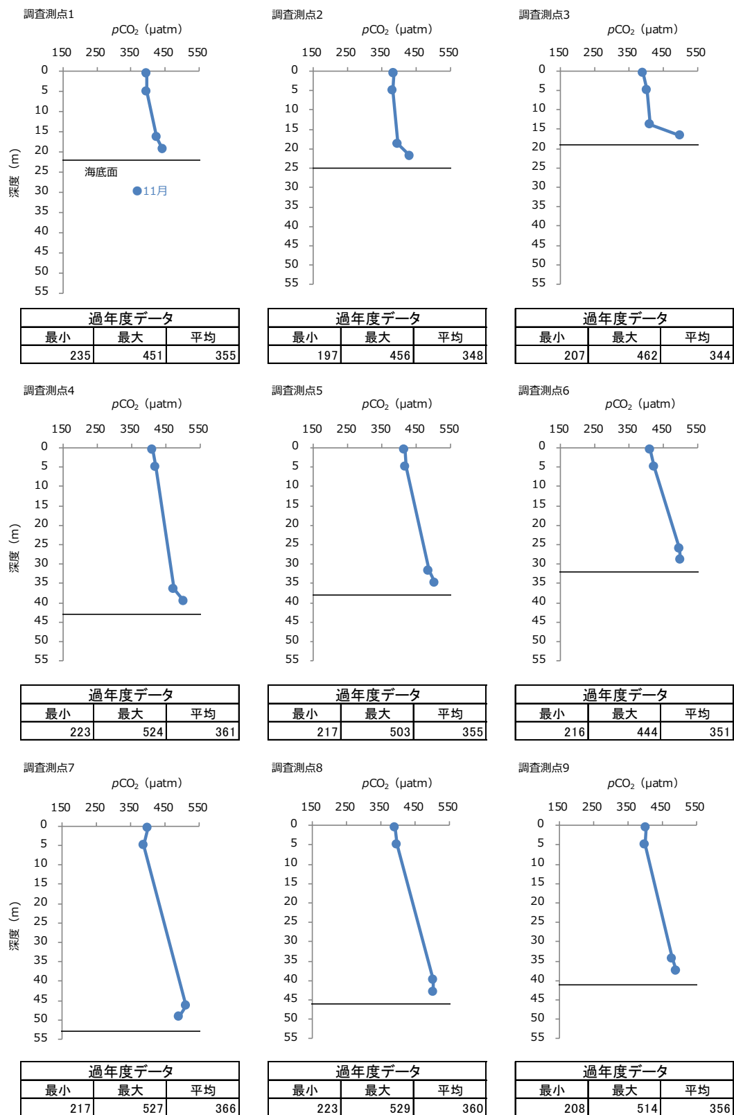
図-14 2021 年度秋季 各調査測点における二酸化炭素分圧 ( p\text{CO}_2 ) の鉛直プロファイル
