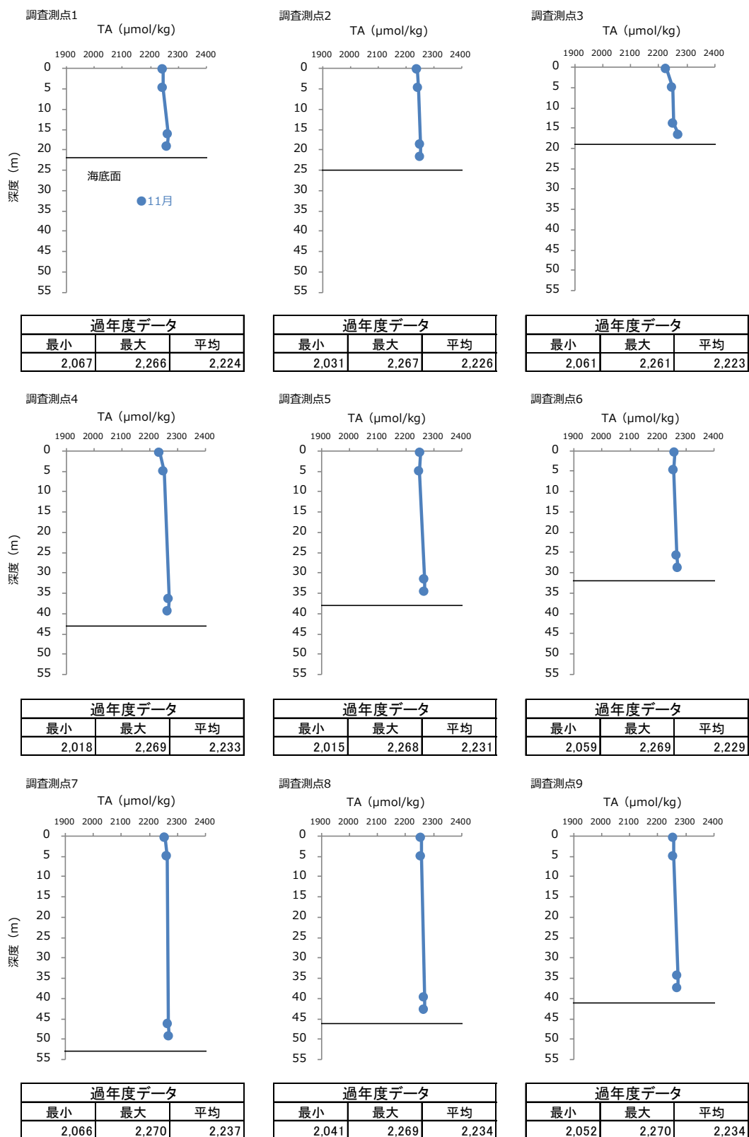
図-8 2021 年度秋季 各調査測点におけるアルカリ度 (TA) の鉛直プロファイル
