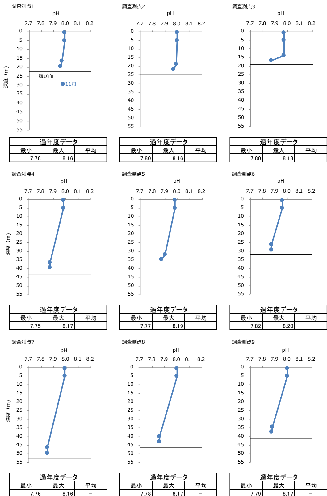
図-12 2021 年度秋季 各調査測点における pH の鉛直プロファイル
