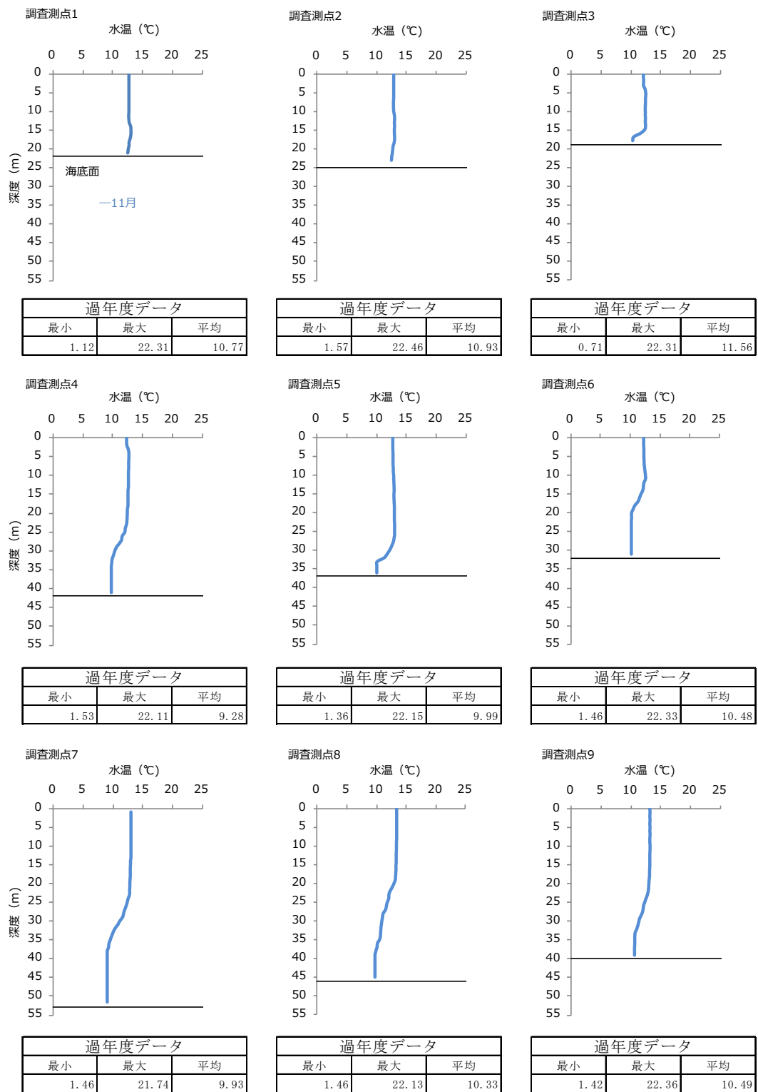
図-2 2021 年度秋季 各調査測点における水温の鉛直プロファイル
