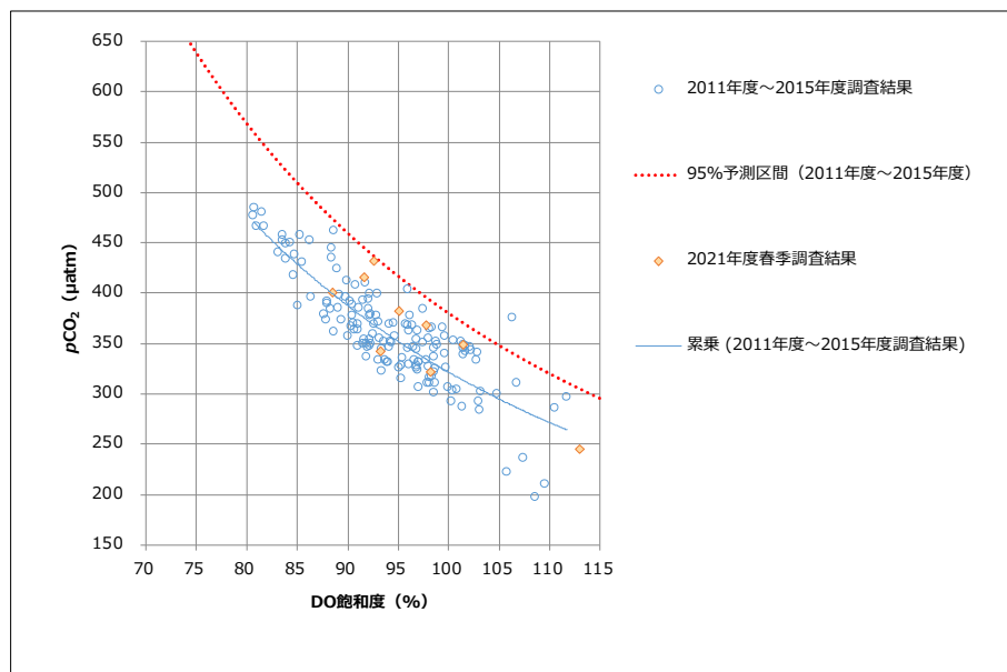
図 5 p\text{CO}_2 と DO 飽和度との関係
