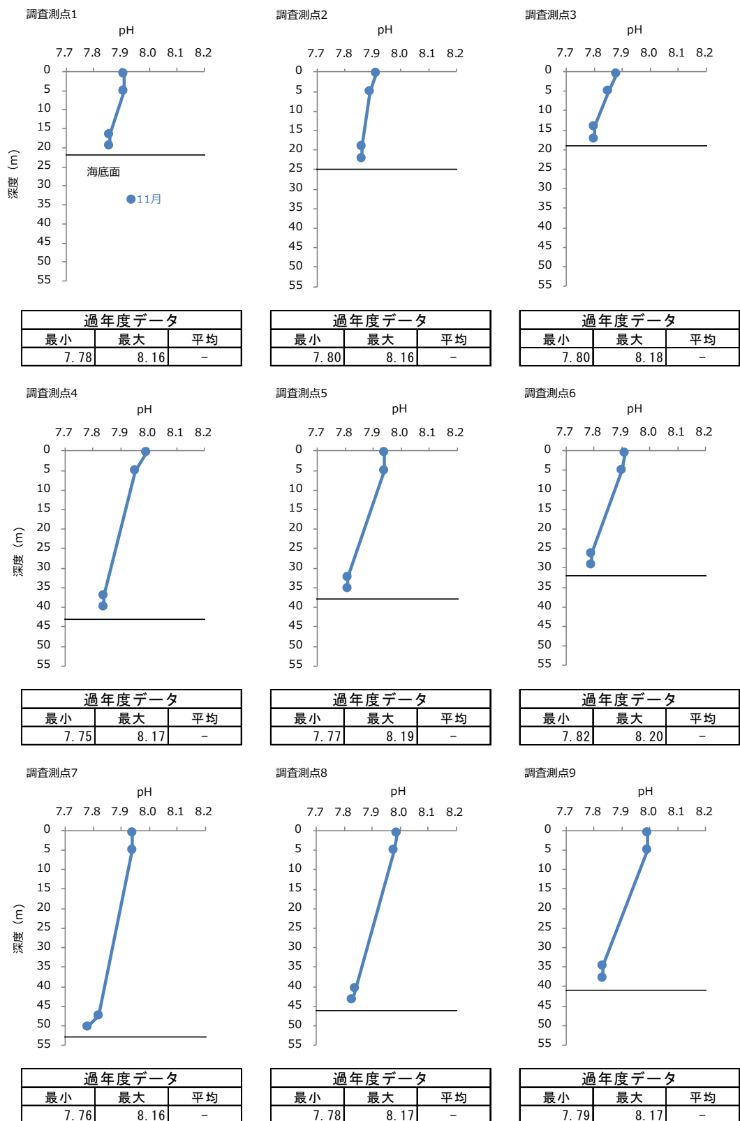
図-12 2023 年度秋季 各調査測点における pH の鉛直プロファイル
