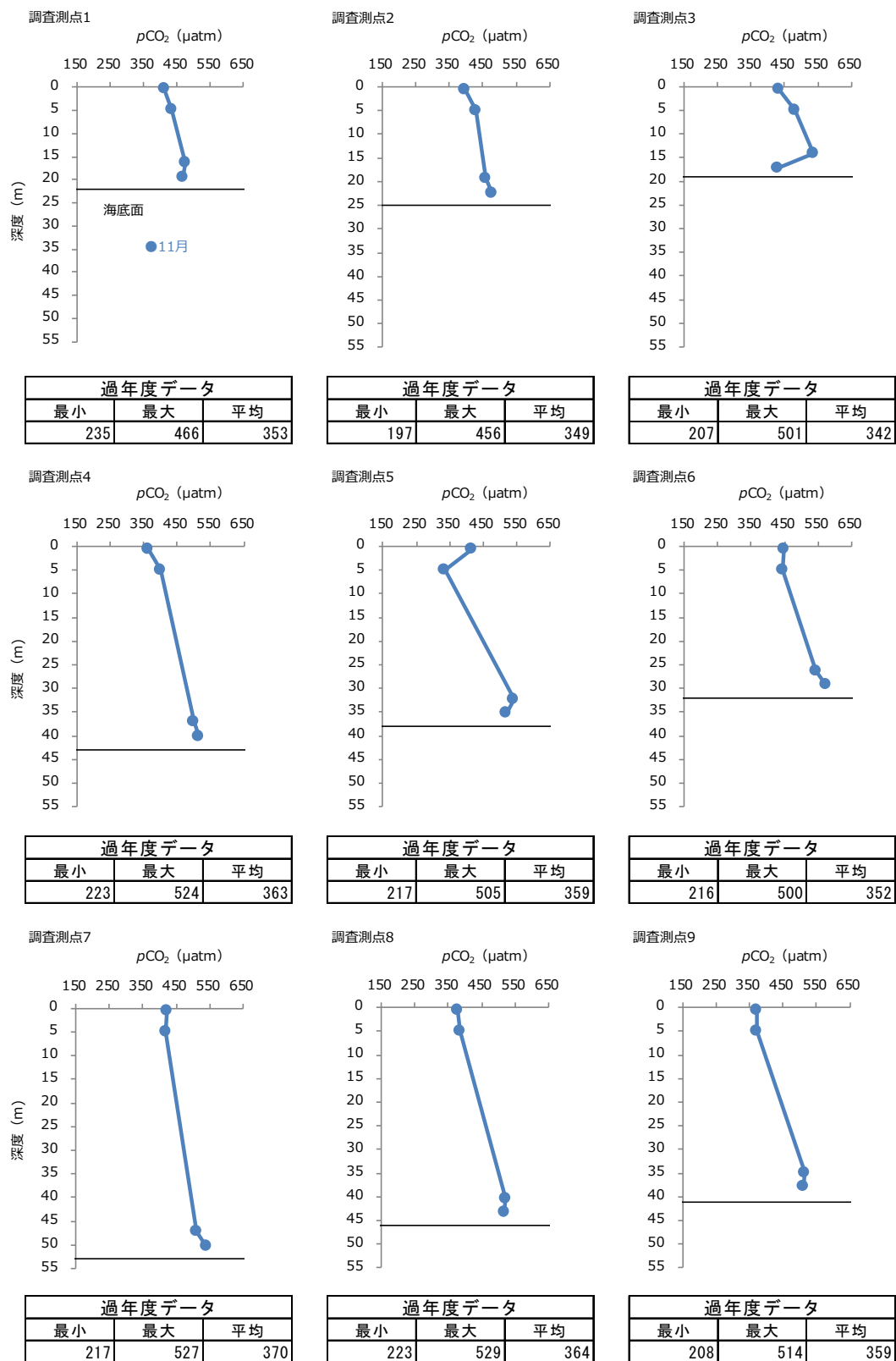
図-14 2023 年度秋季 各調査測点における二酸化炭素分圧 ( pCO_2 ) の鉛直プロファイル
