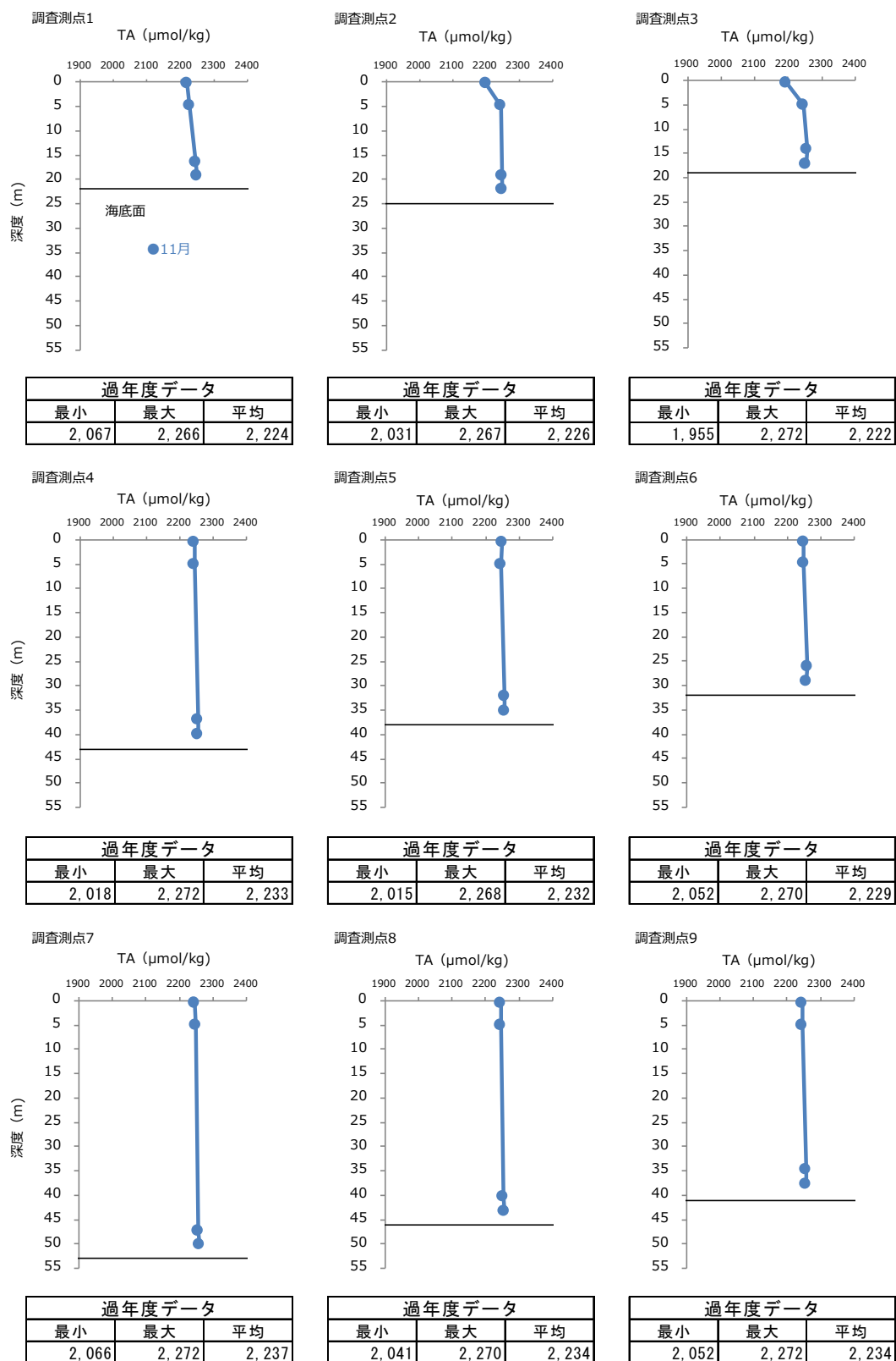
図-8 2023 年度秋季 各調査測点におけるアルカリ度（TA）の鉛直プロファイル
