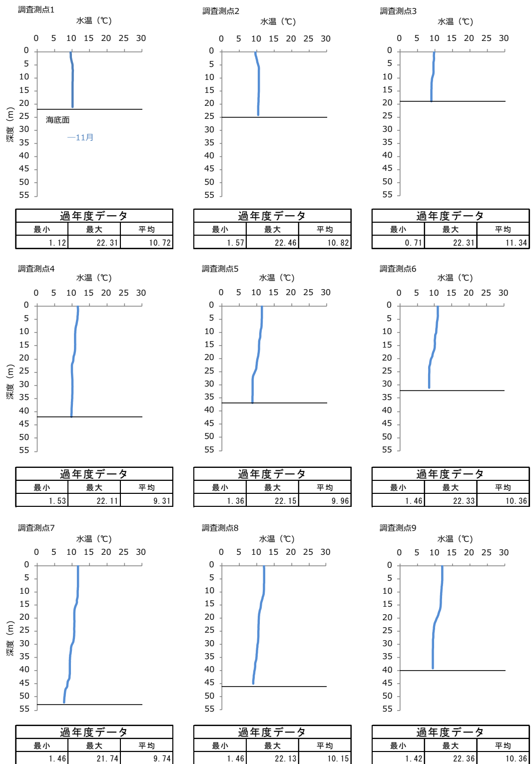
図-2 2023 年度秋季 各調査測点における水温の鉛直プロファイル
