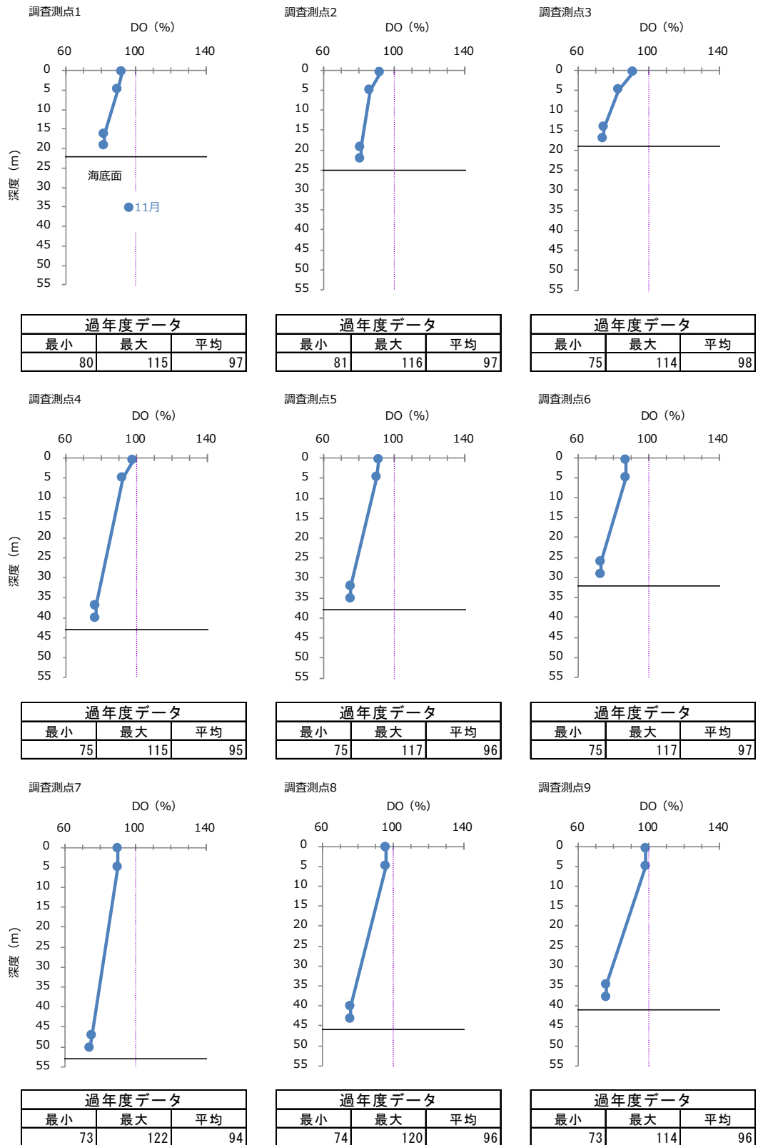
図-16 2023 年度秋季 各調査測点における溶存酸素（DO）飽和度の鉛直プロファイル
