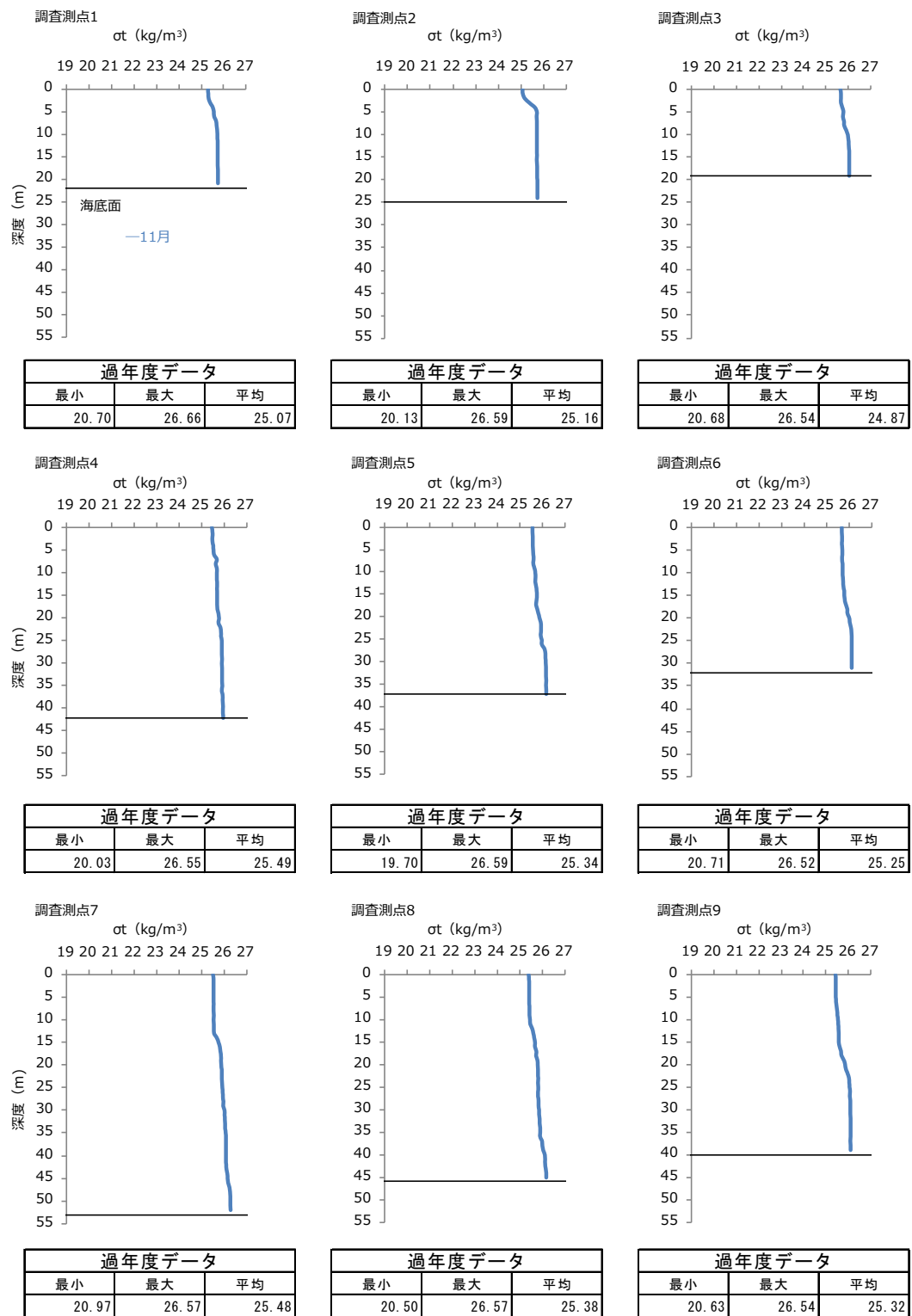
図-6 2023 年度秋季 各調査測点における海水密度（ \sigma_t ）の鉛直プロファイル
