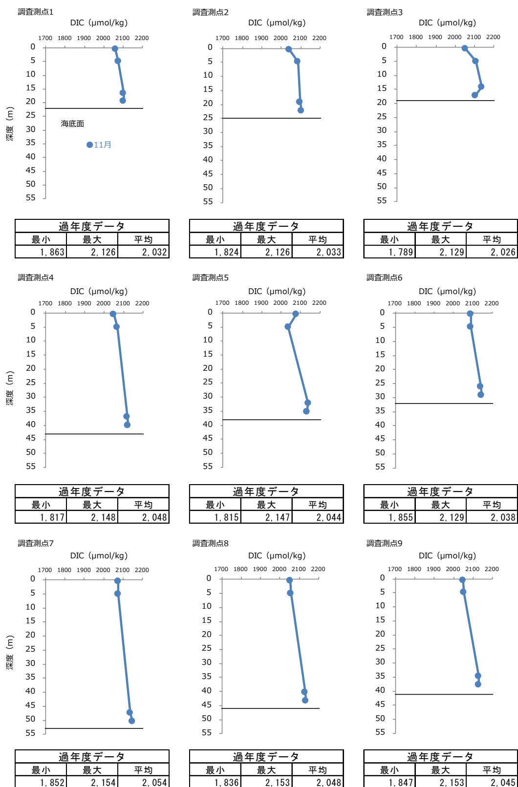
図-10 2023 年度秋季 各調査測点における全炭酸 (DIC) 濃度の鉛直プロファイル
