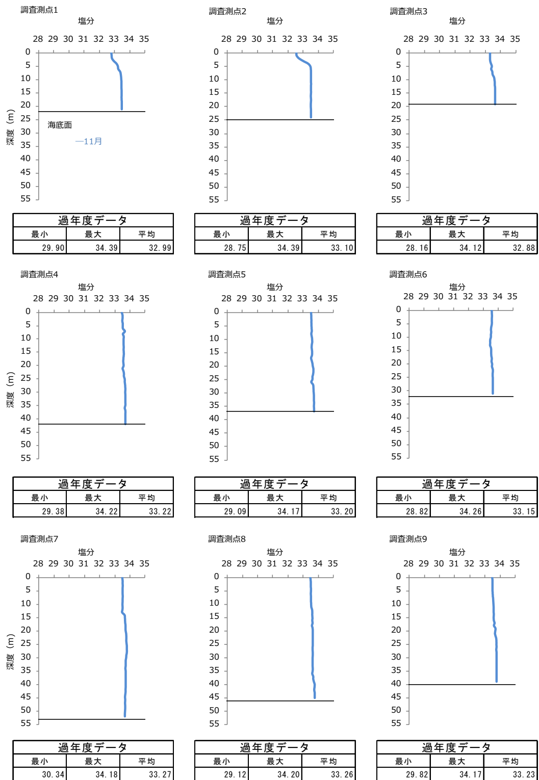
図-4 2023 年度秋季 各調査測点における塩分の鉛直プロファイル
