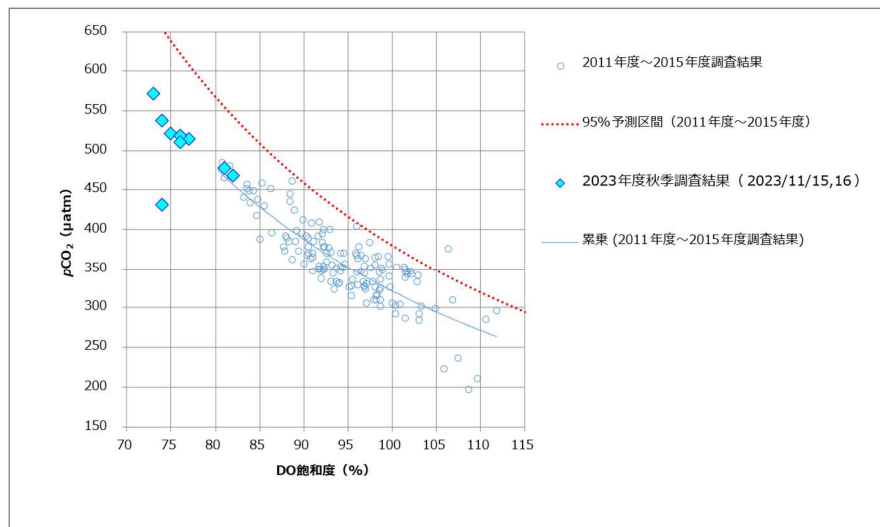
図 2 p\text{CO}_2 と DO 飽和度との関係
