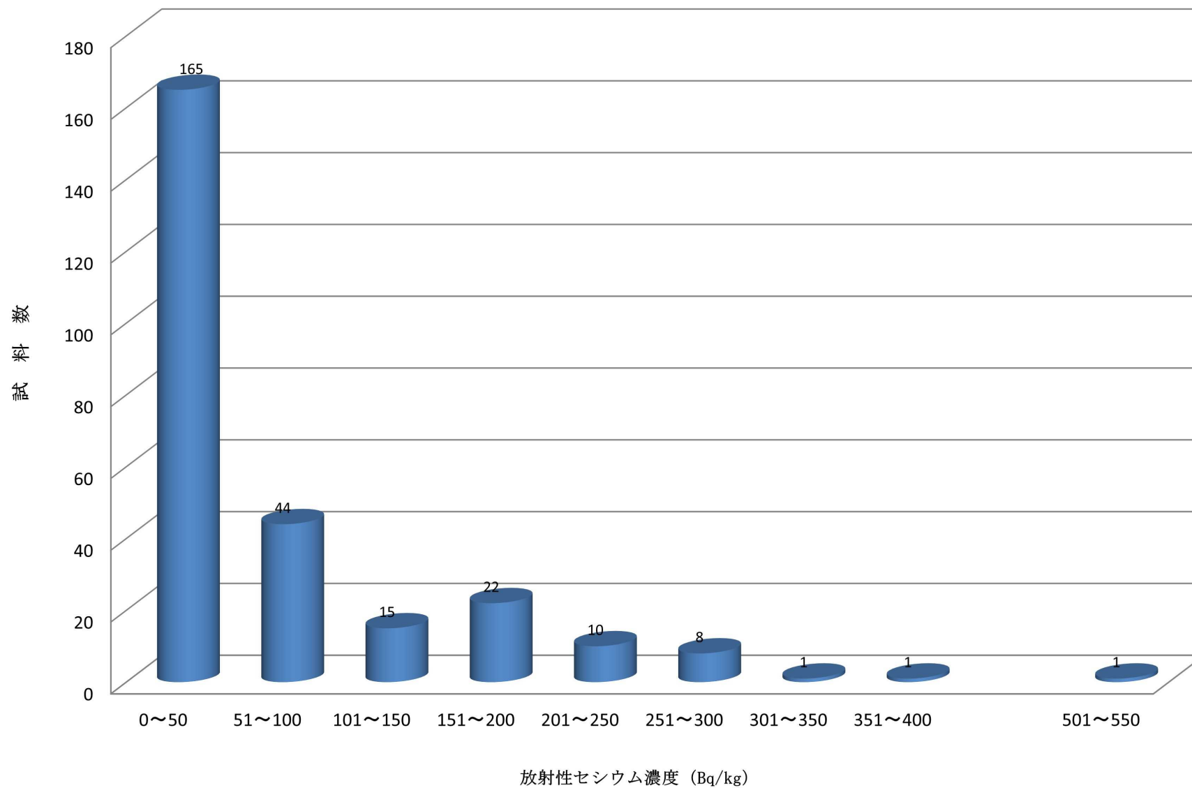
沿岸（底質）の放射性セシウム濃度（50Bq/kg）ごとの頻度（令和5年度）
