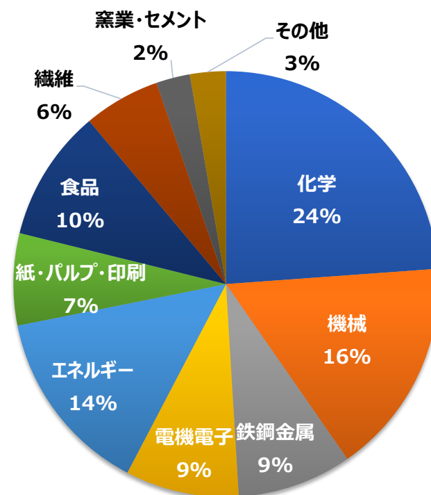
②産業用コージェネレーション業種別発電容量割合（2022年度末）
