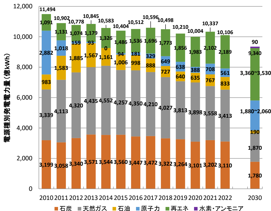
電源種別の発電電力量の推移
