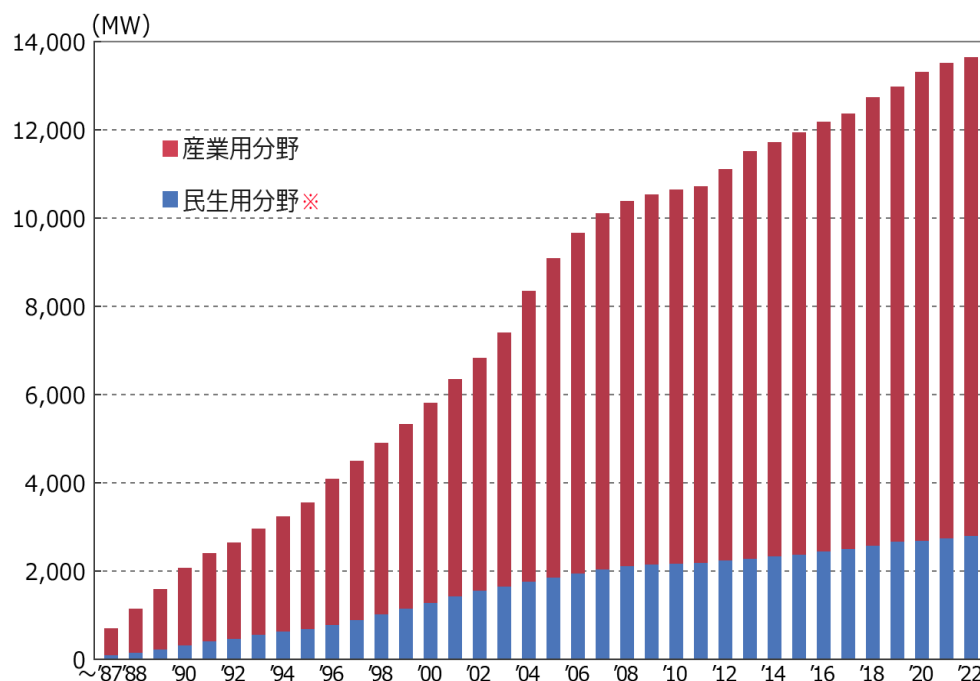
①2022年度末までの業務部門におけるコージェネレーション累積導入容量の推移※
