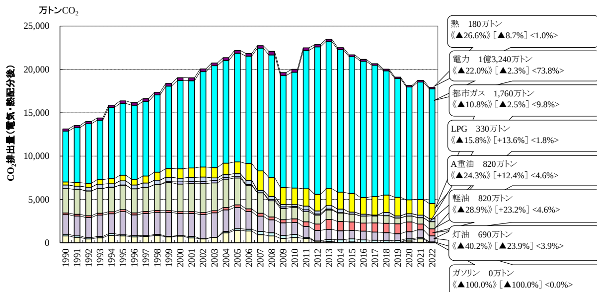
①燃料種別CO 2 排出量
