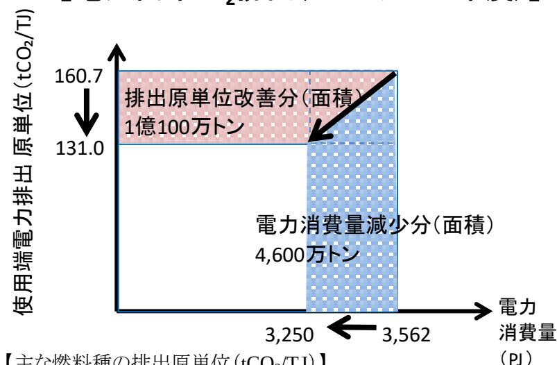
【電力由来CO 2 排出(2013→2022年度)】
