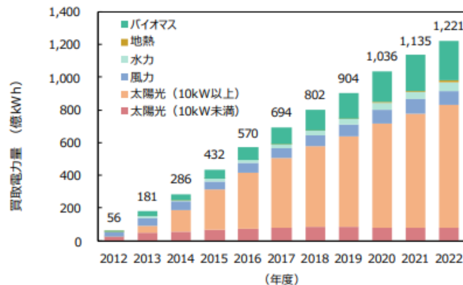
②固定価格買取制度における再生可能エネルギー発電設備を用いた発電電力量の買取実績
