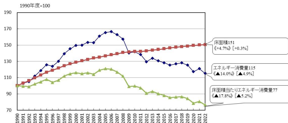
床面積当たりエネルギー消費量
