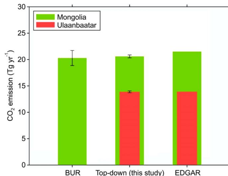
モンゴル国及び首都ウランバートルからの、BUR（左）、GOSAT（中）、公開統計等により算出されたデータベース(EDGAR)による二酸化炭素排出量推計値の比較（Watanabe et al(2023)から一部抜粋。）
