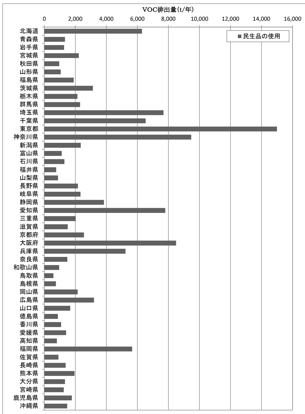
図 7 都道府県別 VOC 排出量の推計結果(令和 2 年度排出量)
