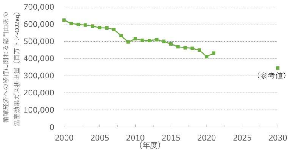
4 図18-1 循環経済への移行に関わる部門由来の温室効果ガス排出量 (環境省作成) 5
