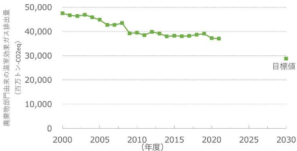
図18-2 廃棄物部門由来の温室効果ガス排出量 (環境省作成)
