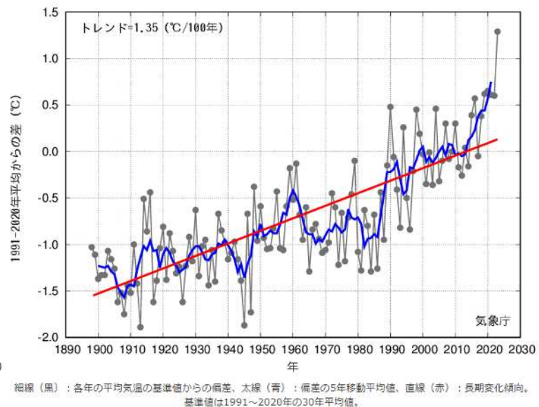
図5 日本の平均気温偏差
