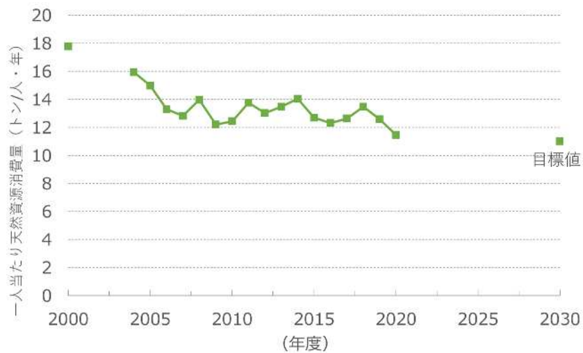
10 図 1 2 一人当たり天然資源消費量の推移（環境省作成）
