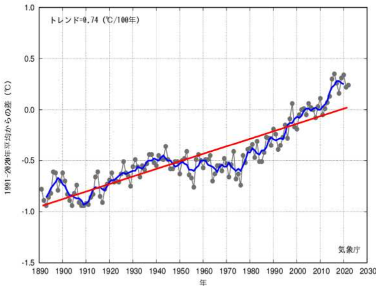
19 図4 世界の平均気温偏差
