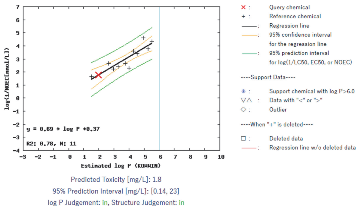
別図 2 KATE2020v4.1 「C_X hydrocarbon unreactive」 回帰式
