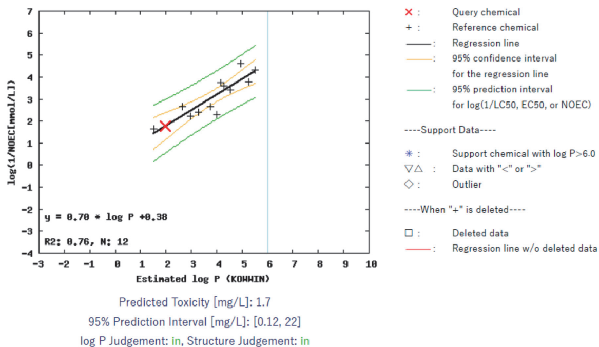
別図 1 KATE2020v4.1 「Cnos_X unreactive Fish Chronic」 回帰式
