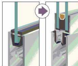
ガラス交換
