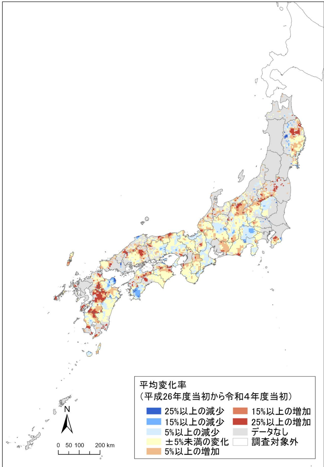
図3 本州以南のニホンジカ密度の平均変化率 (平成26年度(2014年度)から令和4年度(2022年度)の8年間)
