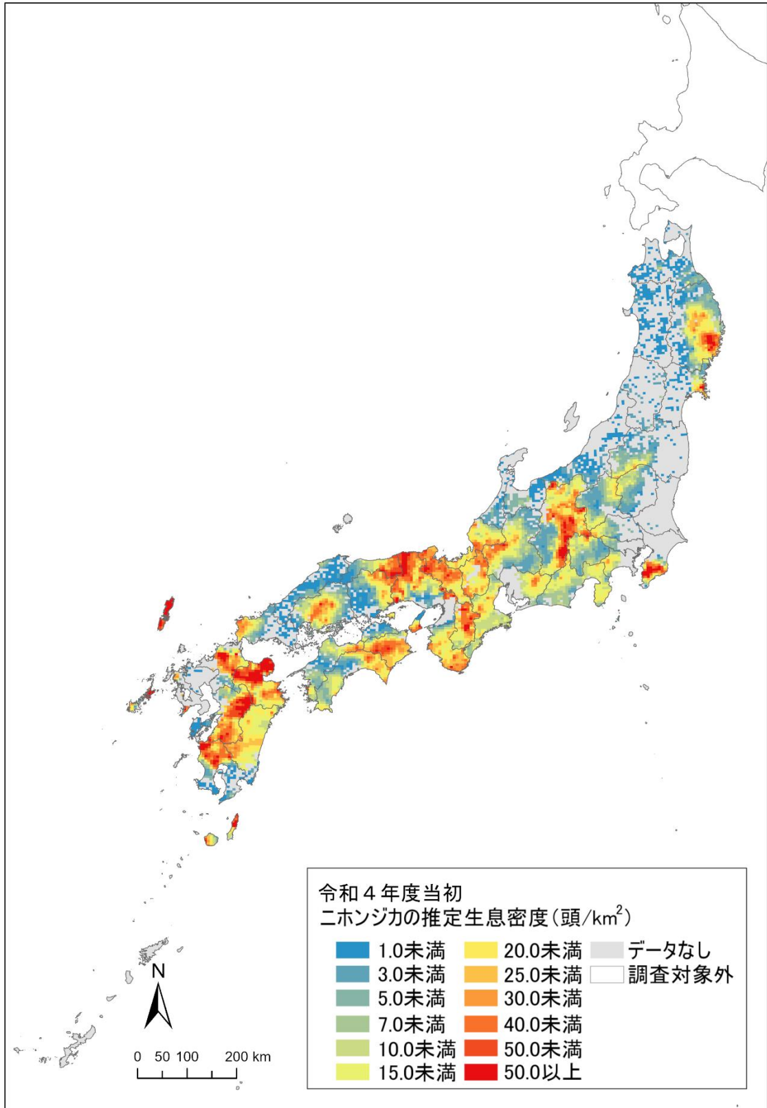
図 1 本州以南のニホンジカ密度分布図(令和 4 年度(2022 年度):中央値)
