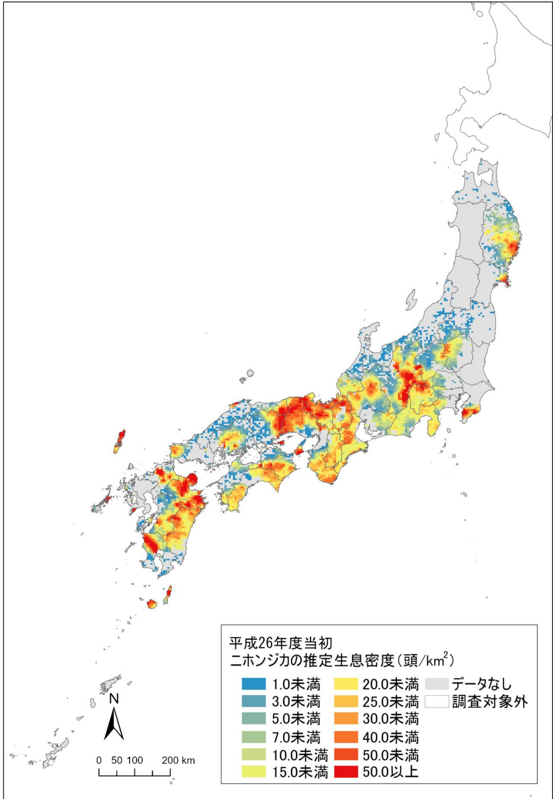
図2 本州以南のニホンジカ密度分布図(平成26年度(2014年度):中央値)
