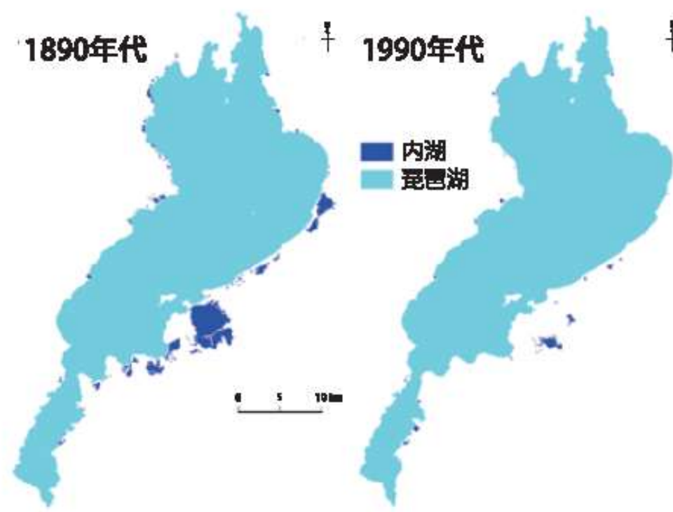
図 1.1.33 明治時代（1890 年代）と平成初期（1990 年代）における琵琶湖と内湖の分布
