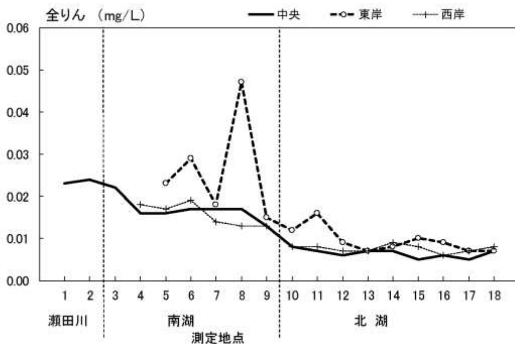
図 1.1.12 琵琶湖における地点別の全磷濃度 (平成 30 年度 (2018 年度) 平均値)
