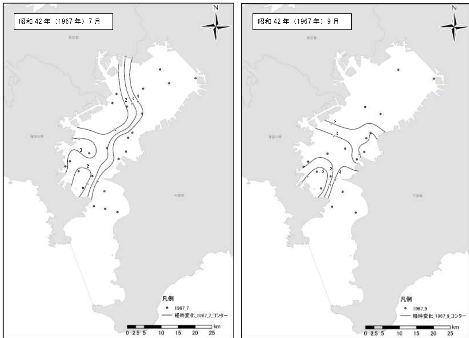
図 1.1.42(13) 昭和30年（1955年）～昭和44年（1969年）の東京湾の底層溶存酸素量の状況
