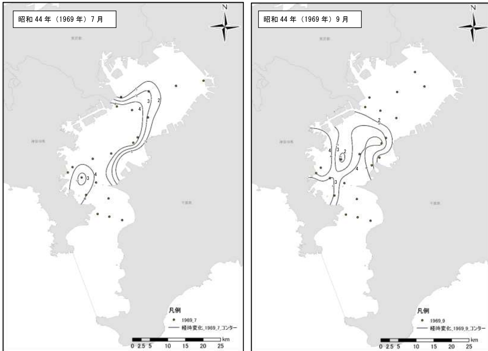
図 1.1.42(15) 昭和30年（1955年）～昭和44年（1969年）の東京湾の底層溶存酸素量の状況
