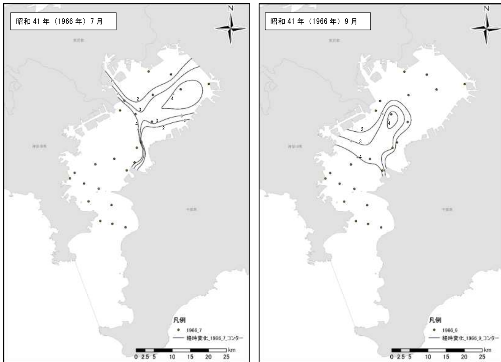
図 1.1.42(12) 昭和 30 年 (1955 年) ~ 昭和 44 年 (1969 年) の東京湾の底層溶存酸素量の状況
