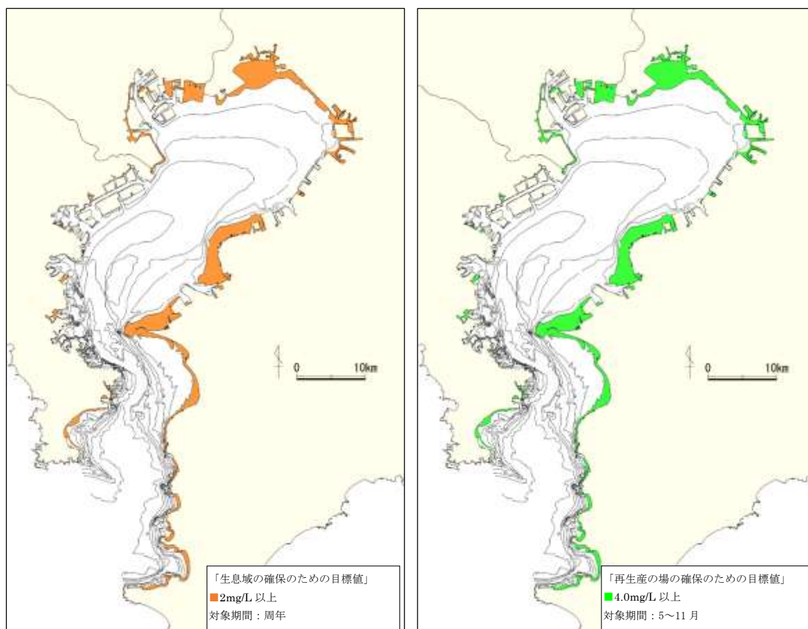
図 1.6.19 ハマグリの生息域及び再生産の場
