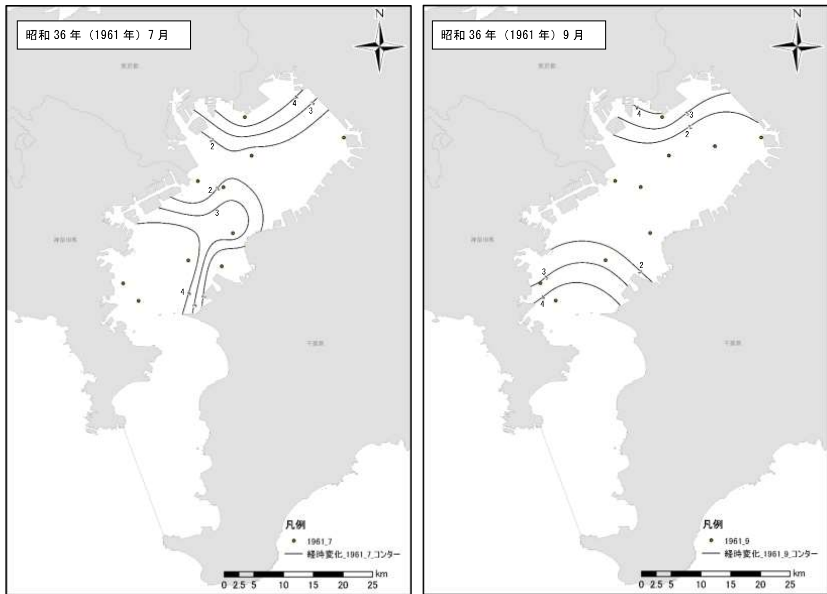
図 1.1.42(7) 昭和 30 年 (1955 年) ~ 昭和 44 年 (1969 年) の東京湾の底層溶存酸素量の状況
