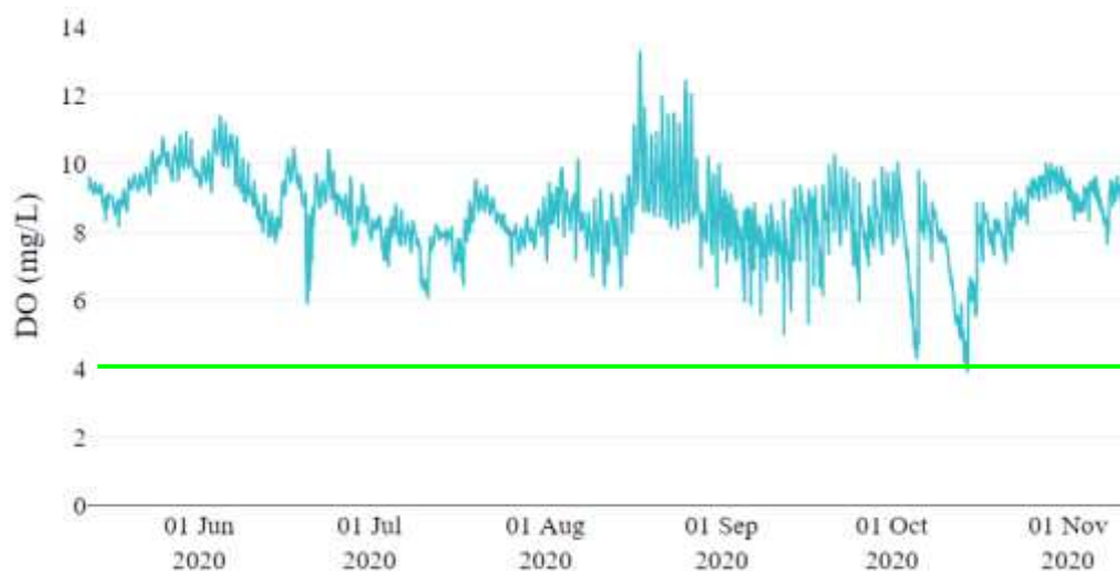
図 1.1.27 唐崎沖中央（6B）における底層溶存酸素量の令和 2 年度（2020 年度）夏季
