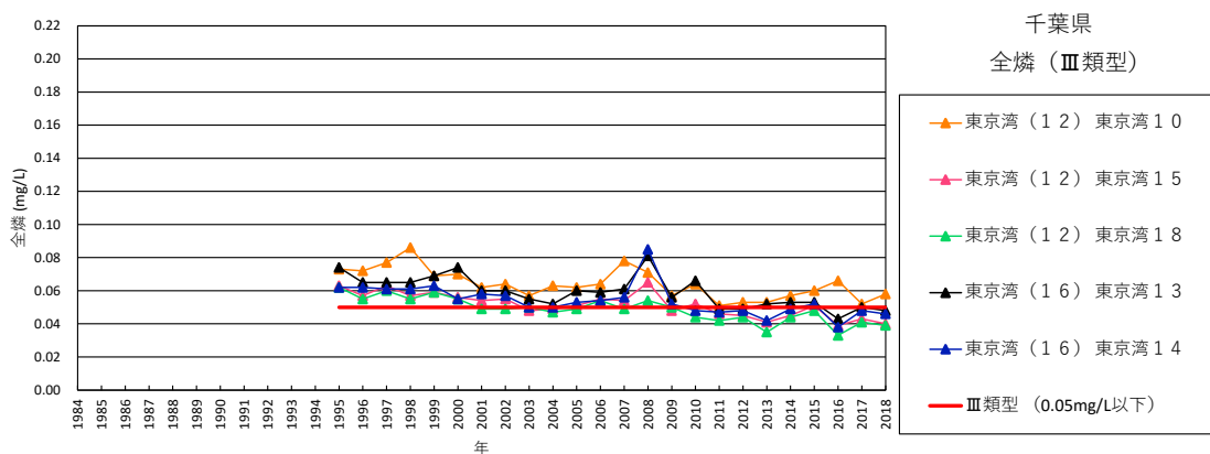
図 1.1.13 東京湾における公共用水域水質測定結果：千葉県（全窒素・全磷）
