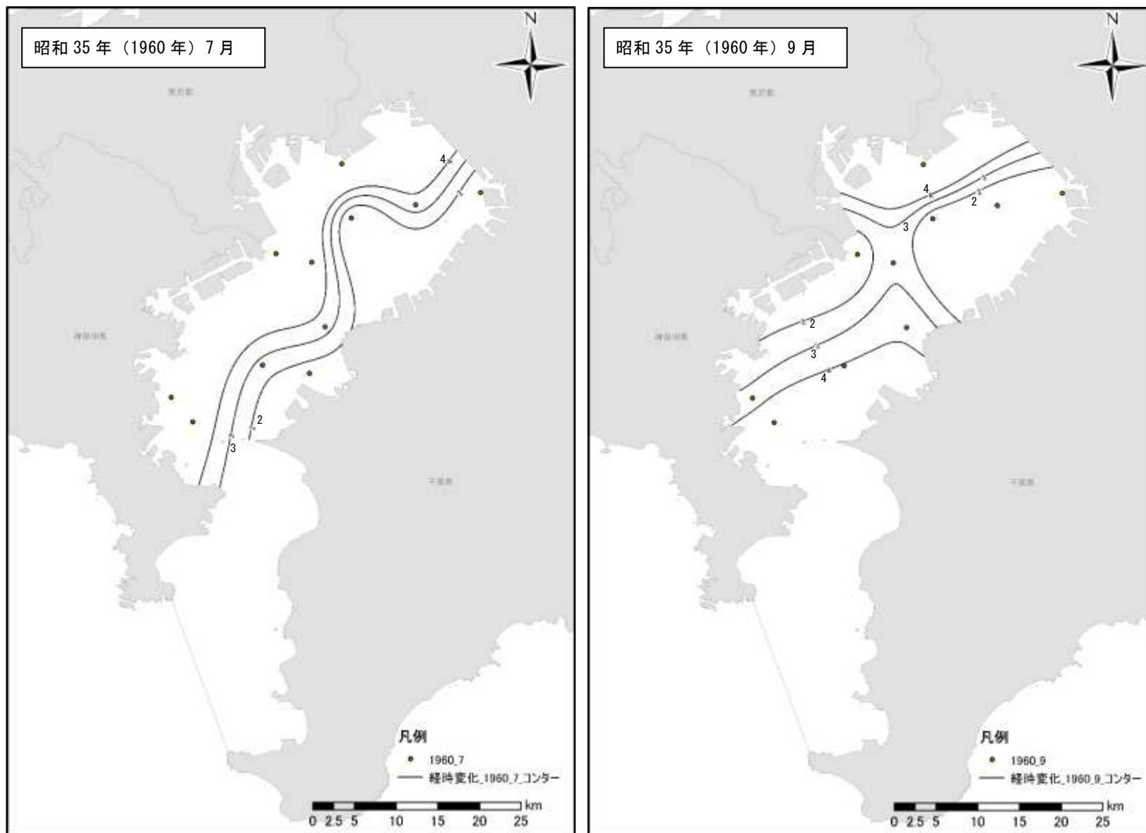
図 1.1.42(6) 昭和30年（1955年）～昭和44年（1969年）の東京湾の底層溶存酸素量の状況
