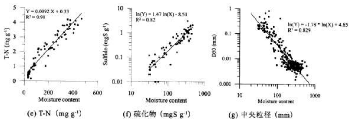
図 1.1.53 含水比と窒素、硫化物、中央粒径の相関関係
