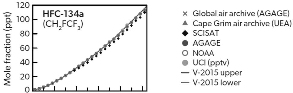
図 2-3-16 海外のネットワークで観測された HFC-134a の濃度変化 各観測ネットワークによる観測結果。
