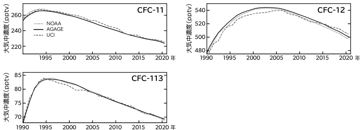
図 2-3-12 海外のネットワークで観測された CFC-11、CFC-12 及び CFC-113 の濃度変化 各観測ネットワークによる観測結果。NOAA による観測結果を実線、AGAGE による観測結果を点線で示している。
