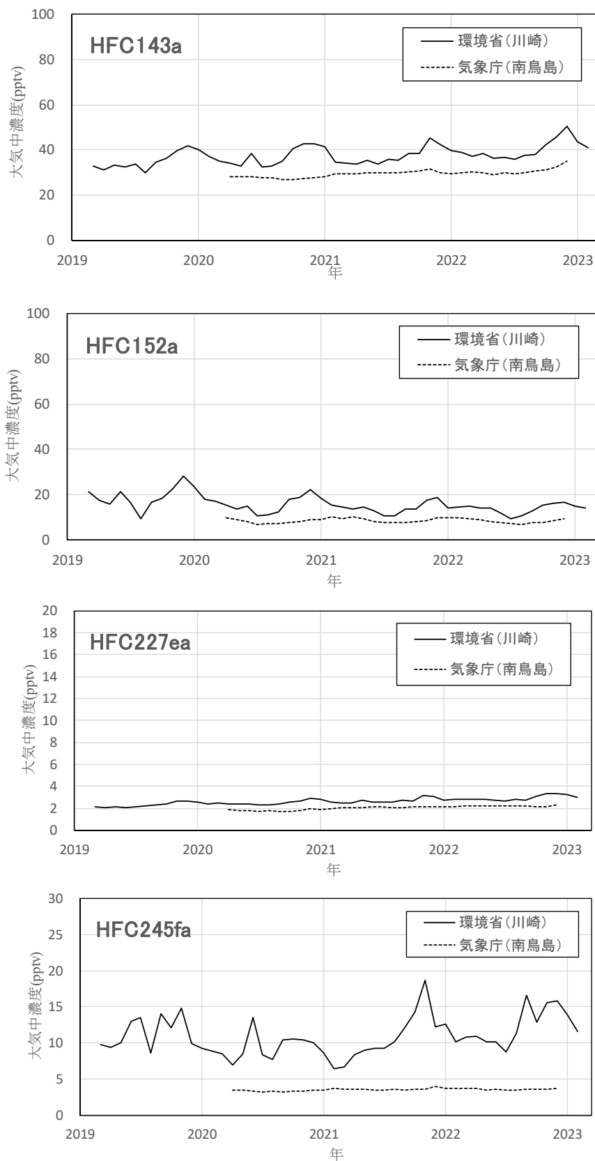
図 2-3-18 川崎市および南鳥島における特定物質等の月別濃度の経年変化（続き） （出典）環境省および気象庁提供データより作図
