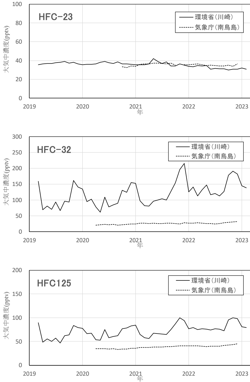
図 2-3-18 川崎市における特定物質等の月別濃度の経年変化（続き）
