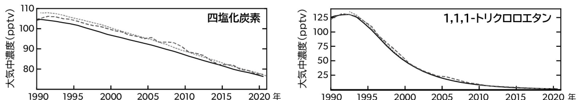
図 2-3-13 海外のネットワークで観測された四塩化炭素及び 1,1,1-トリクロロエタンの濃度変化 各観測ネットワークによる観測結果。NOAA による観測結果を実線、AGAGE による観測結果を点線で示している。
