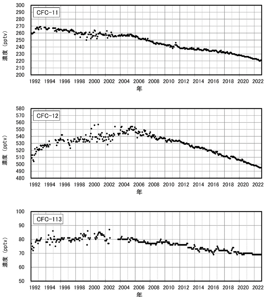
図2-3-10 岩手県大船渡市綾里における大気中のクロロフルオロカーボン類濃度の経年変化 綾里における大気中のCFC-11（上）、CFC-12（中）、CFC-113（下）の地上での月平均濃度（測定結果を月平均したもの）の経年変化を示す。なお、データのない期間は、主に観測機器の更新や校正作業のための欠測である。また、観測精度を向上させるため、2003年9月から放射線源を用いた電子捕獲型検出器（ECD）を搭載したガスクロマトグラフを導入したことにより、観測濃度データのばらつきがそれ以前と比較して少なくなっている。※図④参照。図④では、水色で表している。（出典）気象庁提供
