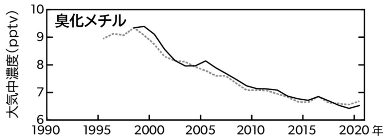
図 2-3-17 海外のネットワークで観測された臭化メチルの濃度変化
