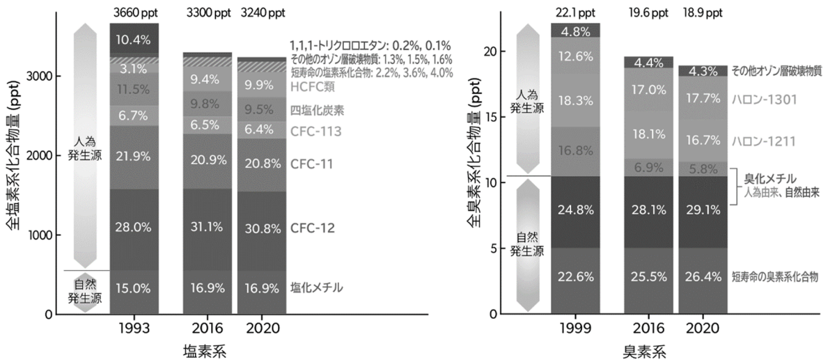
図 2-1-1 1993、1999、2016年及び2020年の成層圏中の塩素・臭素の主要な起源物質 大気中のガスの濃度の単位として「1兆分の1」(ppt)を使用している。1pptは、1兆個の大気分子が存在する中に着目するガス分子が1個の割合で存在することを示す。 (出典) Scientific Assessment of Ozone Depletion: 2022 (WMO, 2022)
