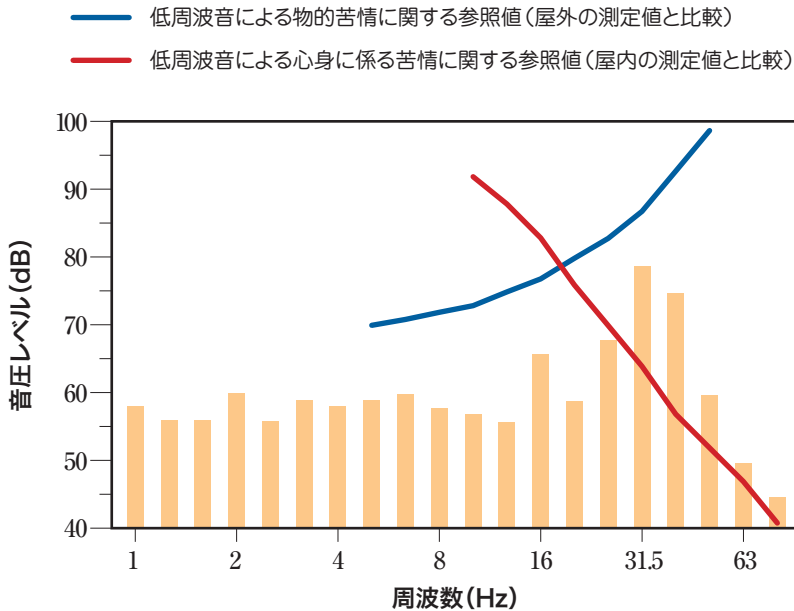
低周波音の測定例と参照値との比較
