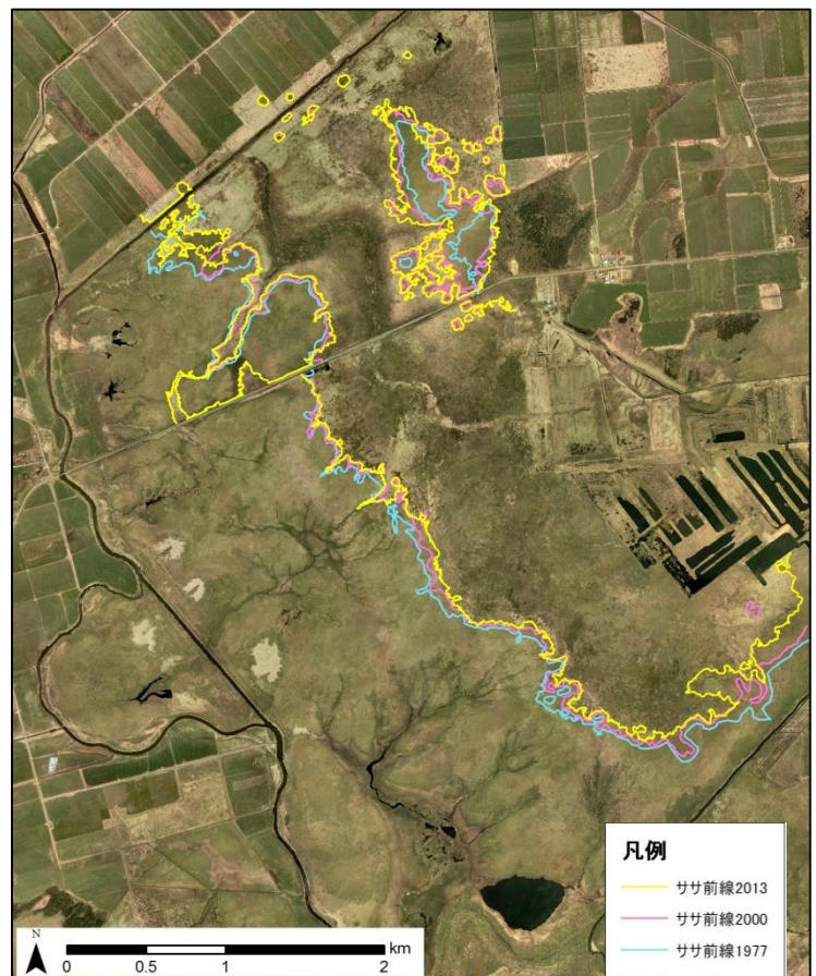
図 5-6 ササ生育地の変化(ササ前線)
