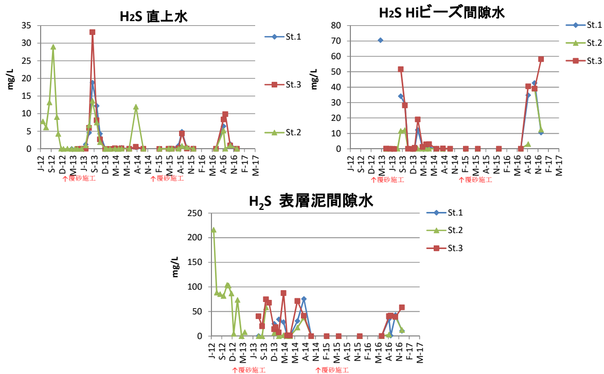
図3. 細井沖浚渫産地の硫化水素濃度.
