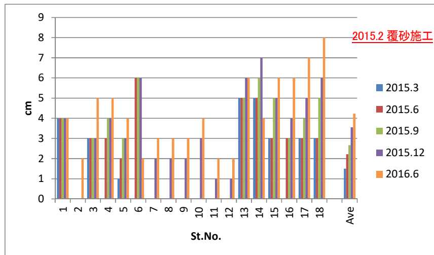
図2. 細井沖浚渫産地の堆積物厚.
