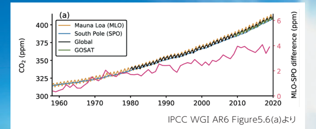
IPCC第6次評価報告書に掲載された GOSATの観測結果 (2009年から始まる緑色の線がGOSATの観測結果)
