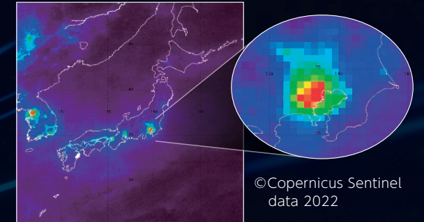
ヨーロッパの衛星によるNO 2 観測結果 (左)日本周辺、(右)東京付近 赤い部分がNO 2 排出量の大きい地点 GOSAT-GWではCO 2 も同時に観測します
