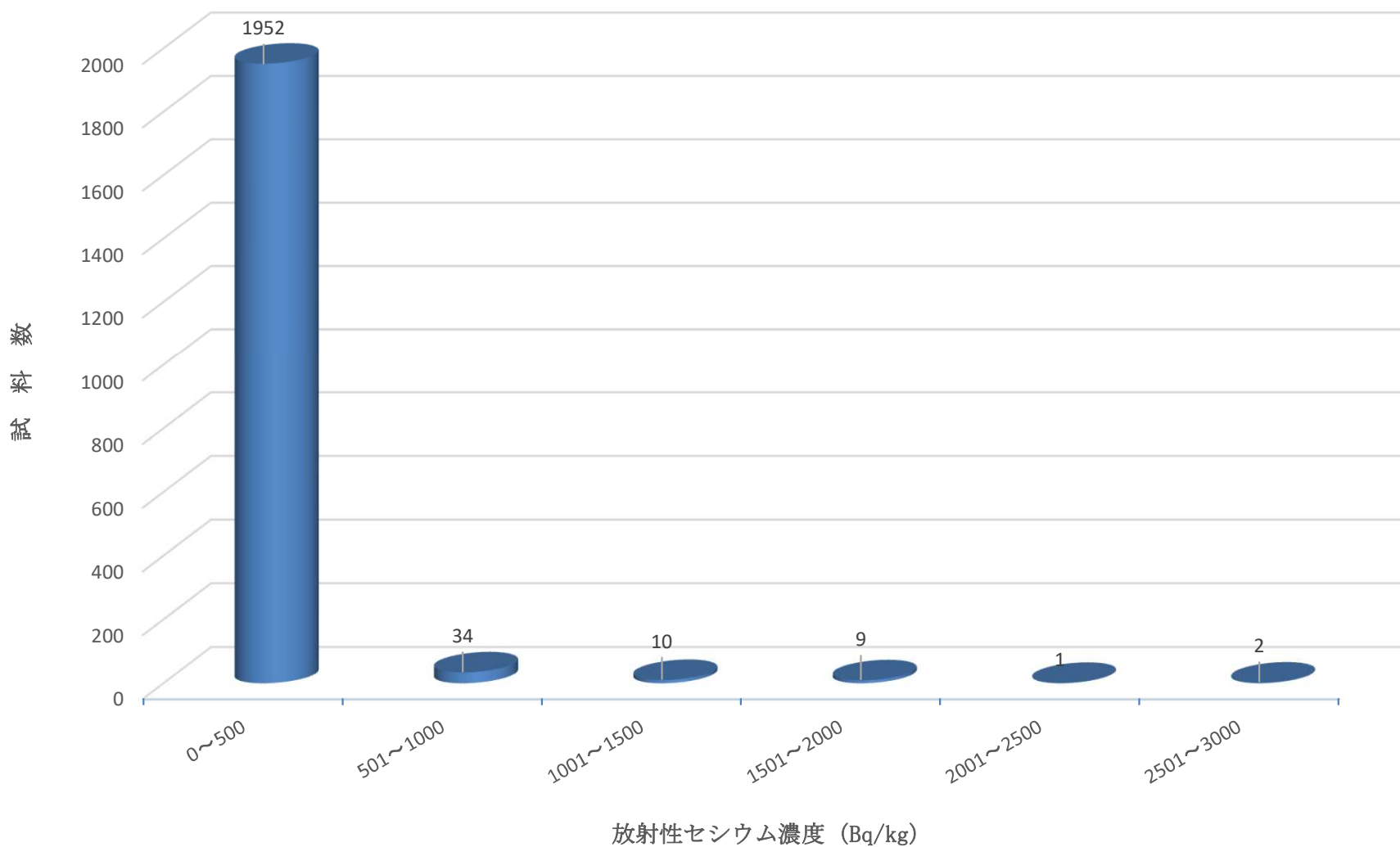
河川（底質）の放射性セシウム濃度（500Bq/kg）ごとの頻度（令和4年度）
